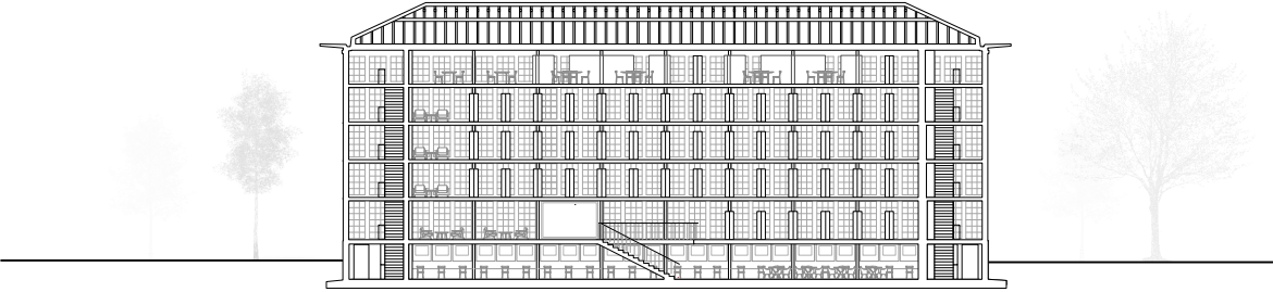
Schnitt B
