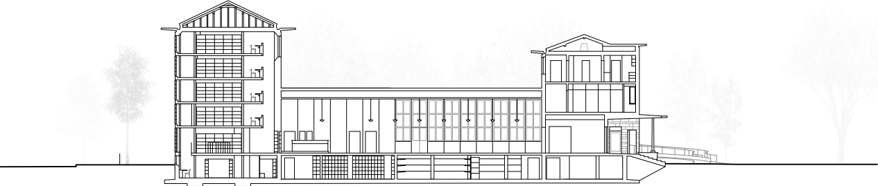
Schnitt D
