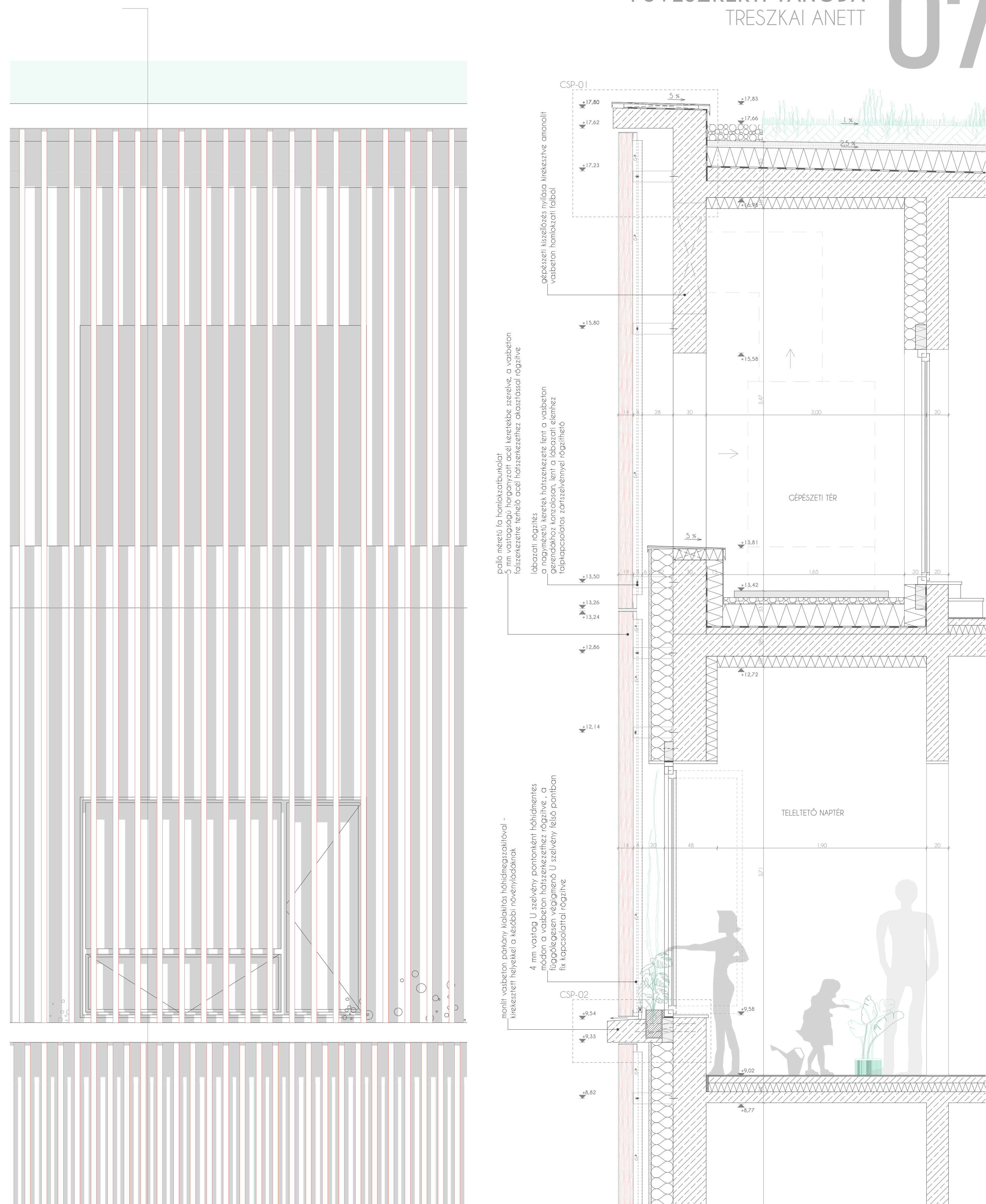
TORONY ÉPÜLET_HOMLOKZATI RÉSZLETRAJZ 1:20
