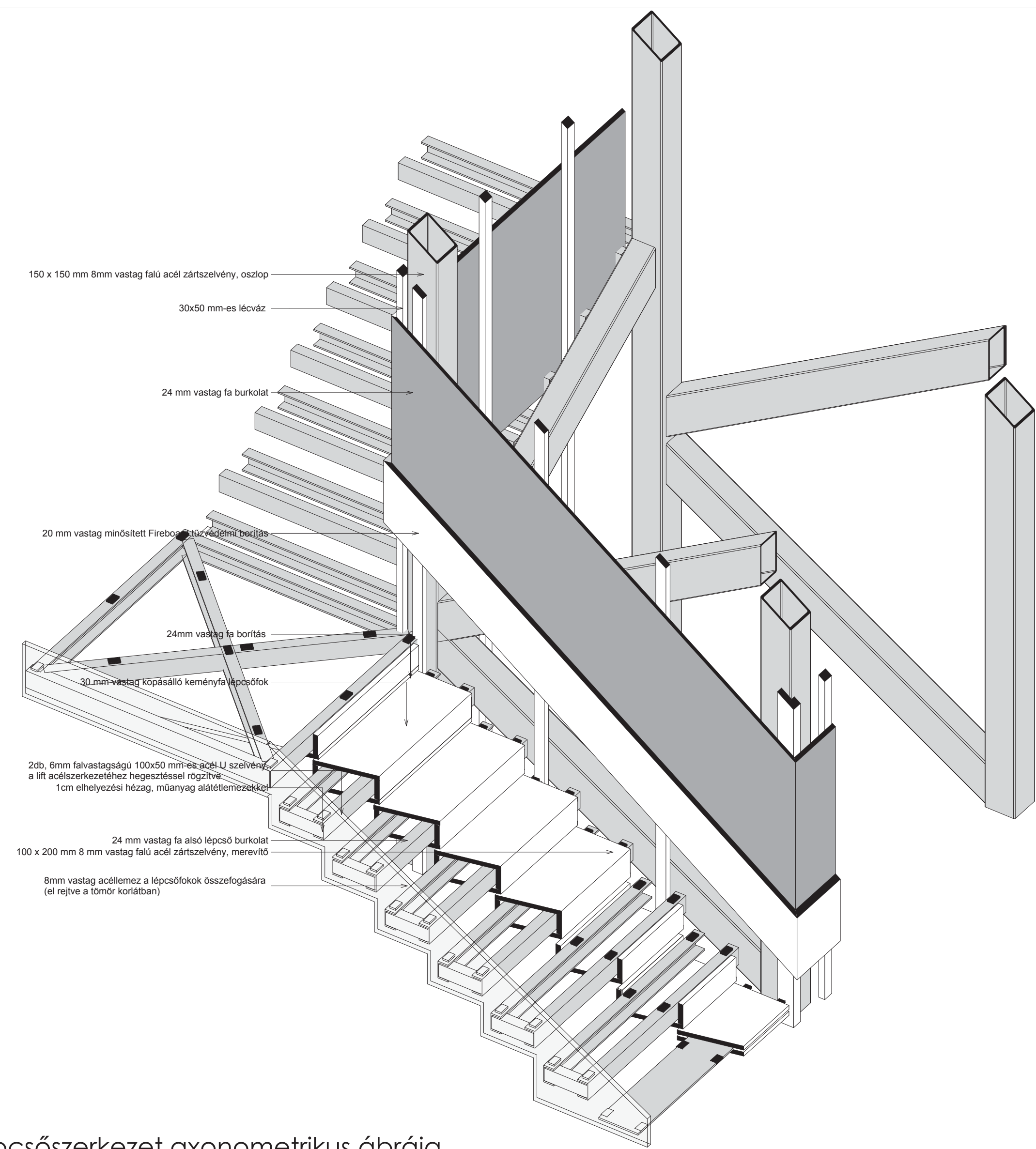
Acél lépcsőszerkezet axonometrikus ábrája
