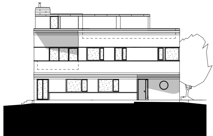
FATADA SUD
