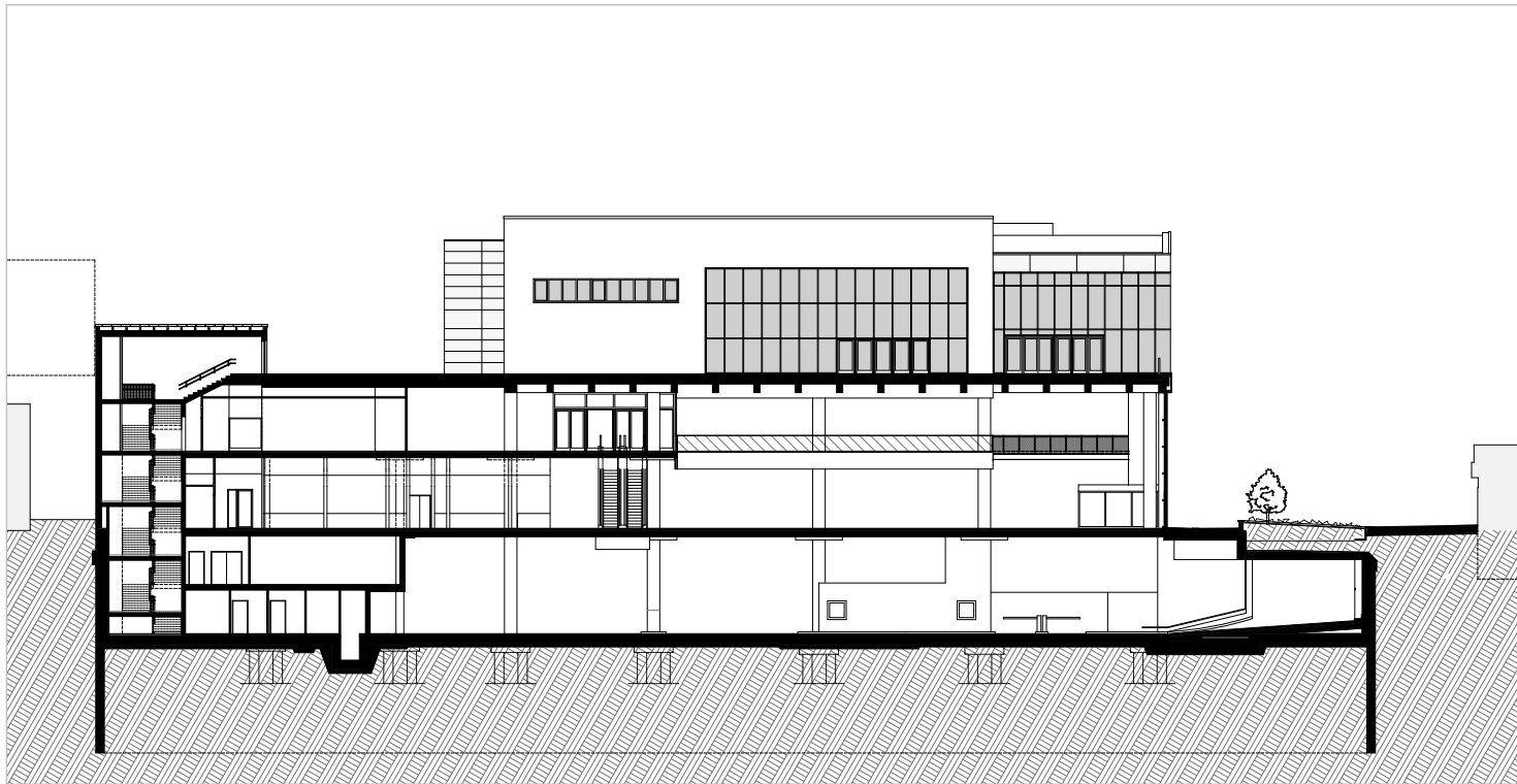
I-I metszet - rendezvényközpont déli homlozat / I-I section - Cultural Center south elevation
