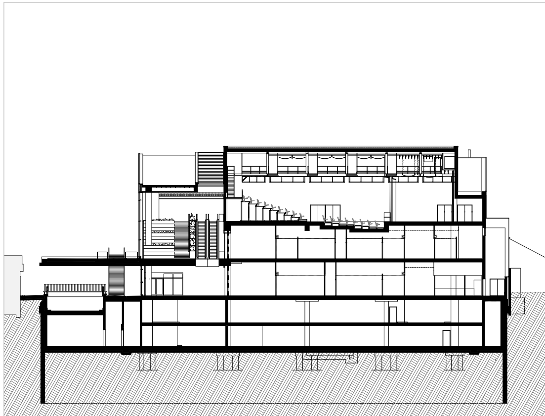
K-K metszet - U2 északi homlozat / K-K section - U2 north elevation
