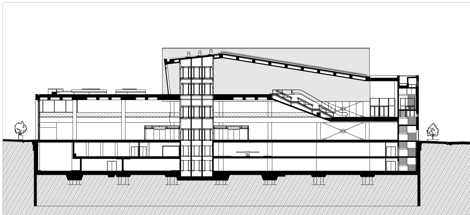
E-E metszet / E-E section
