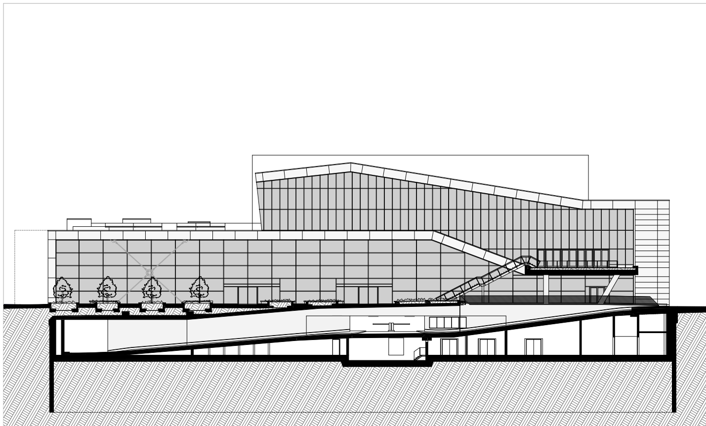
Szent István téri homlokzat garázs rámpa metszettel / Szent István square elevation with garage ramp section
