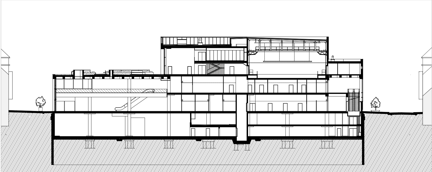
D-D metszet / D-D section
