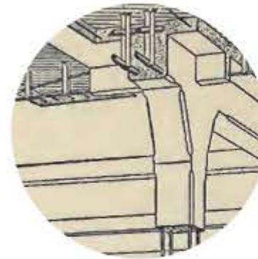
Vasbeton födém
