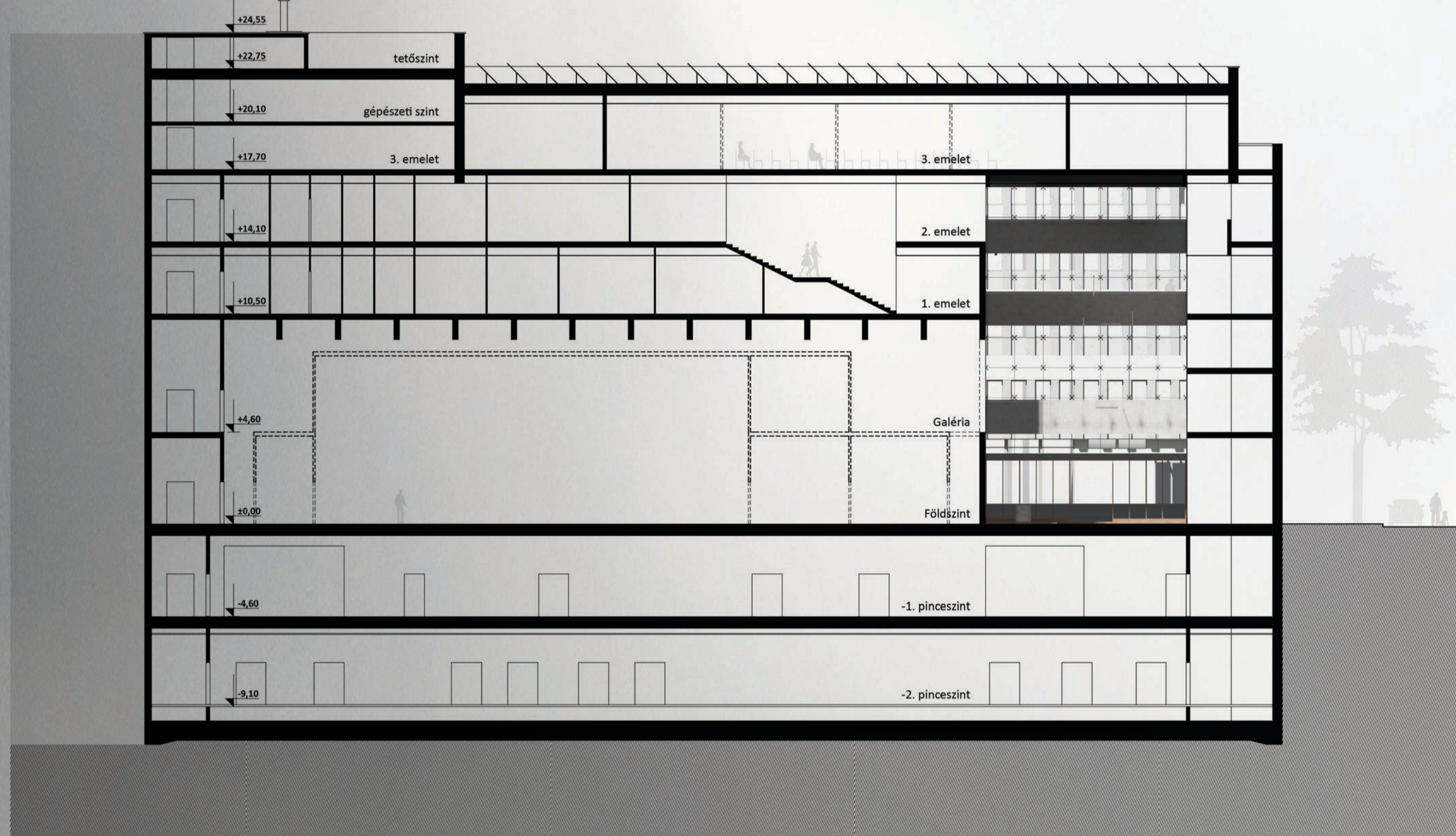
C-C metszet M 1:200
