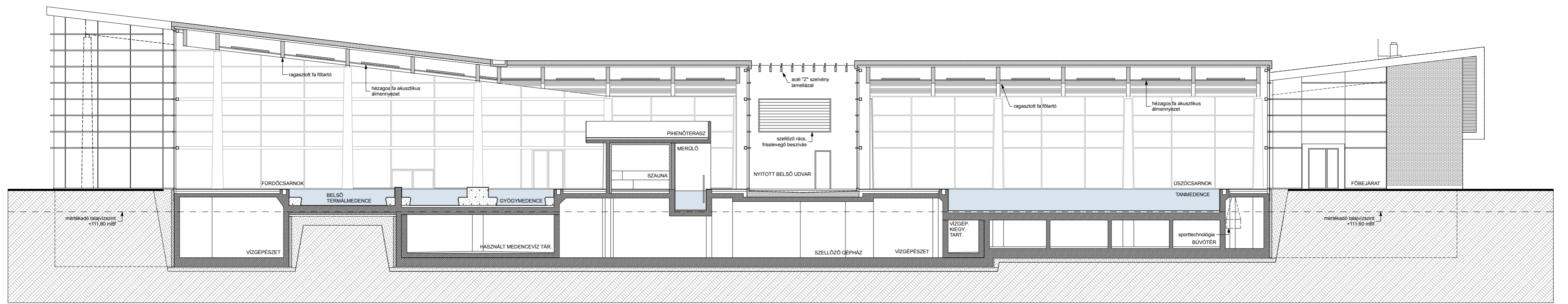
EE METSZET
