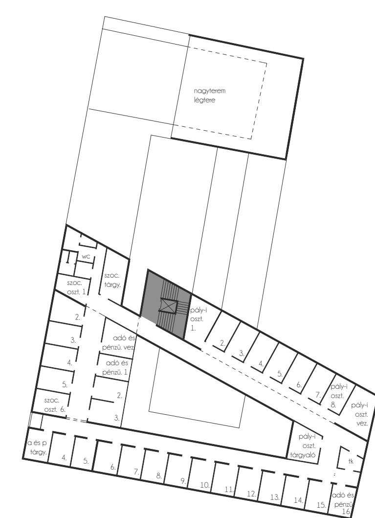
1. EMELETI ALAPRAJZ
