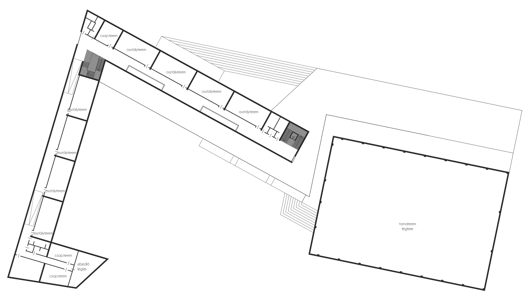
1. EMELETI ALAPRAJZ
