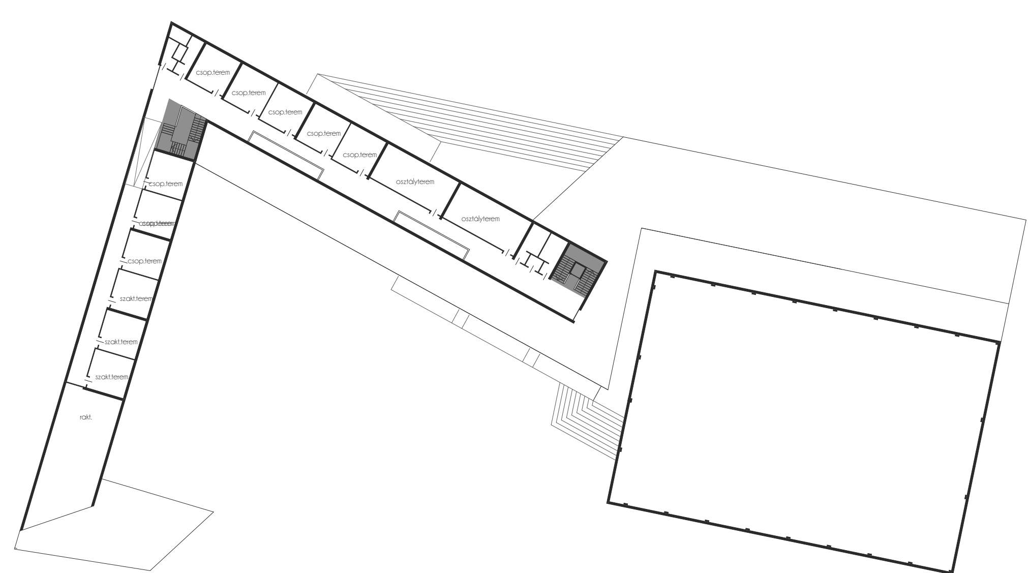
2. EMELETI ALAPRAJZ
