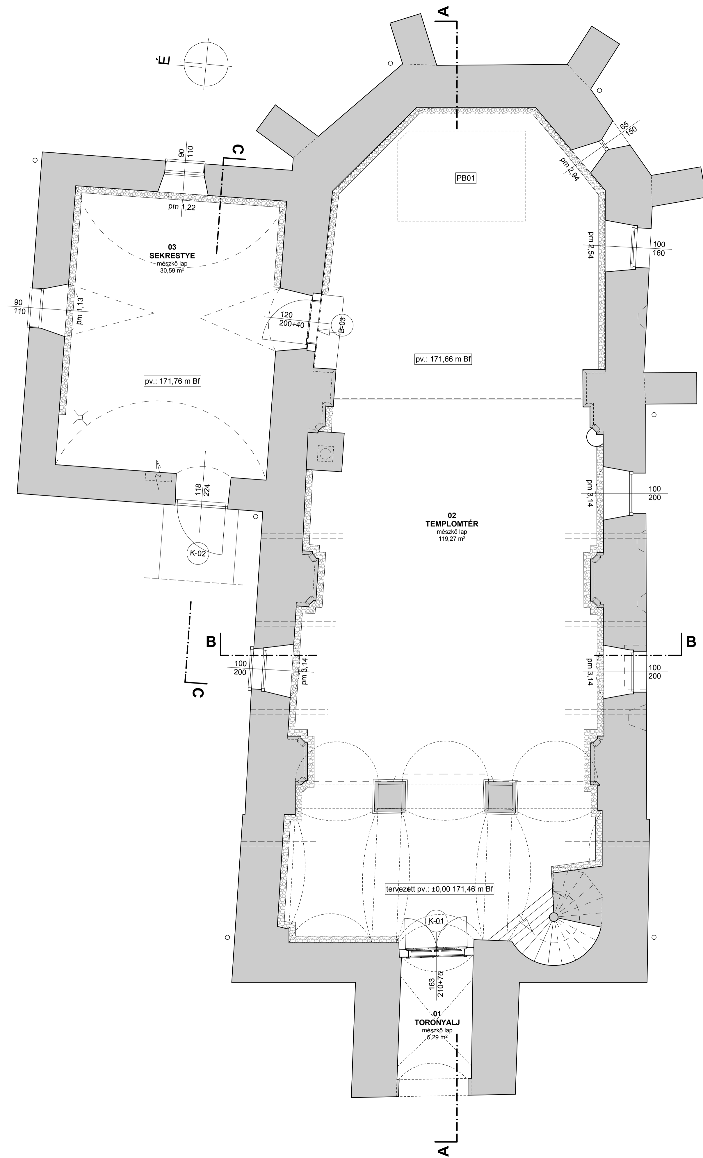
Földszint tervezett alaprajza M 1:50
