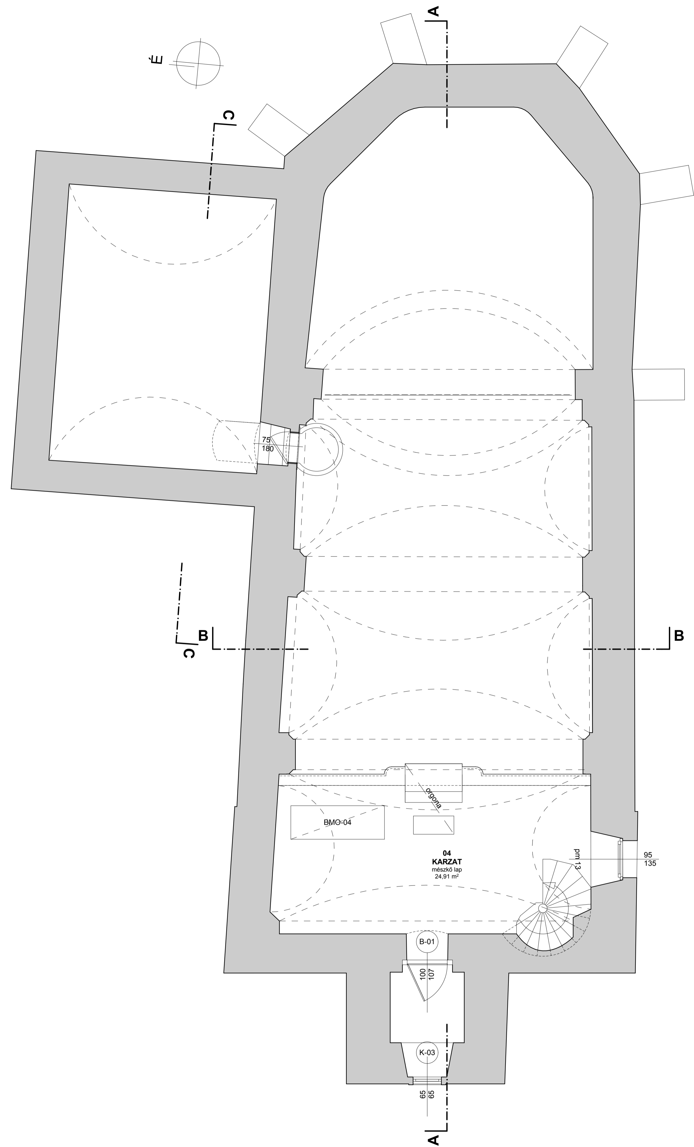
Karzat tervezett alaprajza M 1:50
