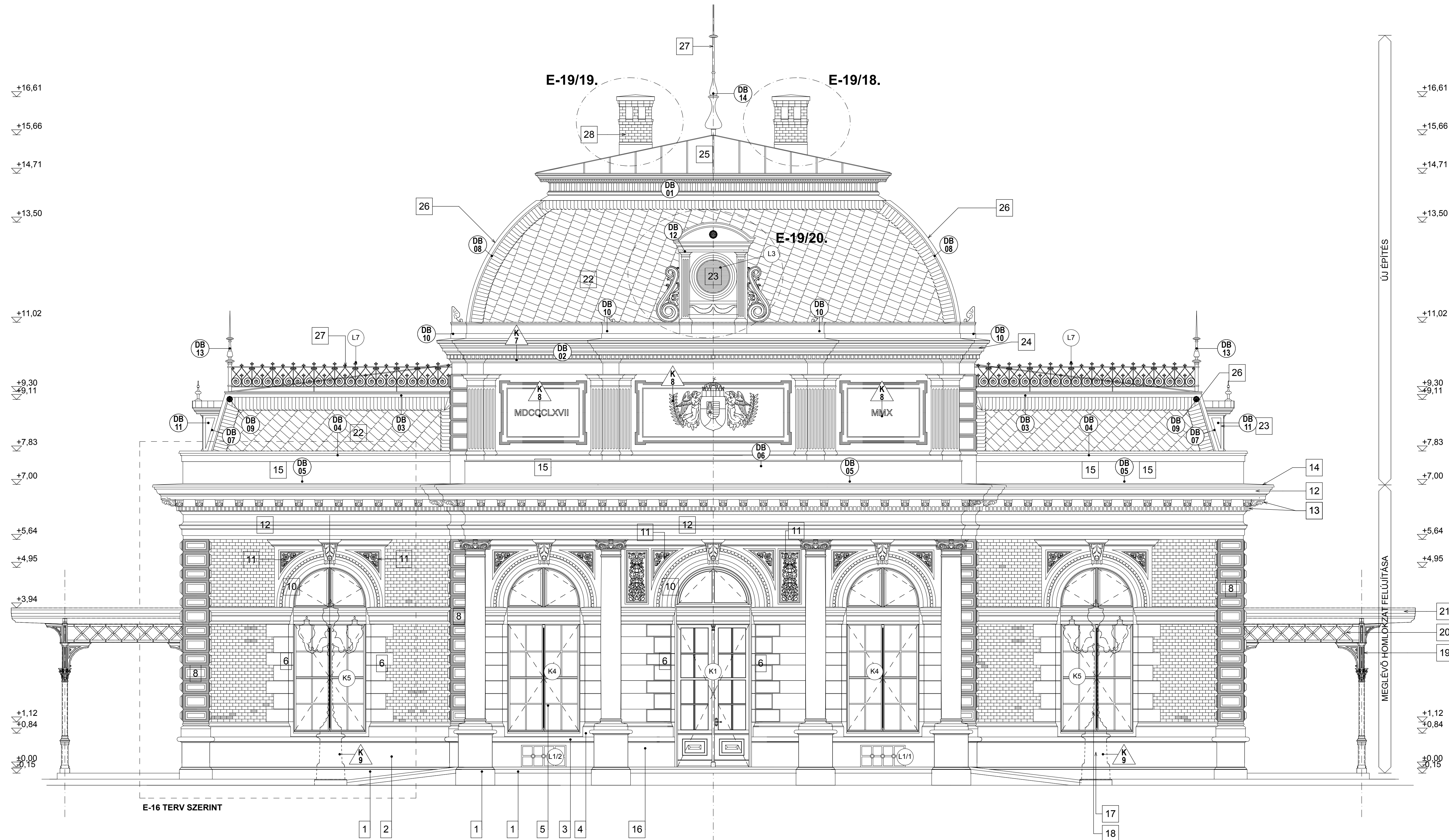
NYUGATI HOMLOKZAT M=1:50
