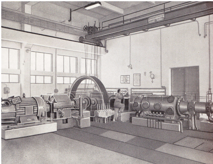
Nagynyomású levegőkompreszor
