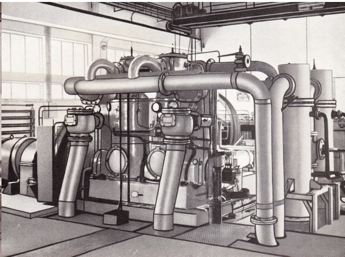
Kisnyomású levegőkompreszor
