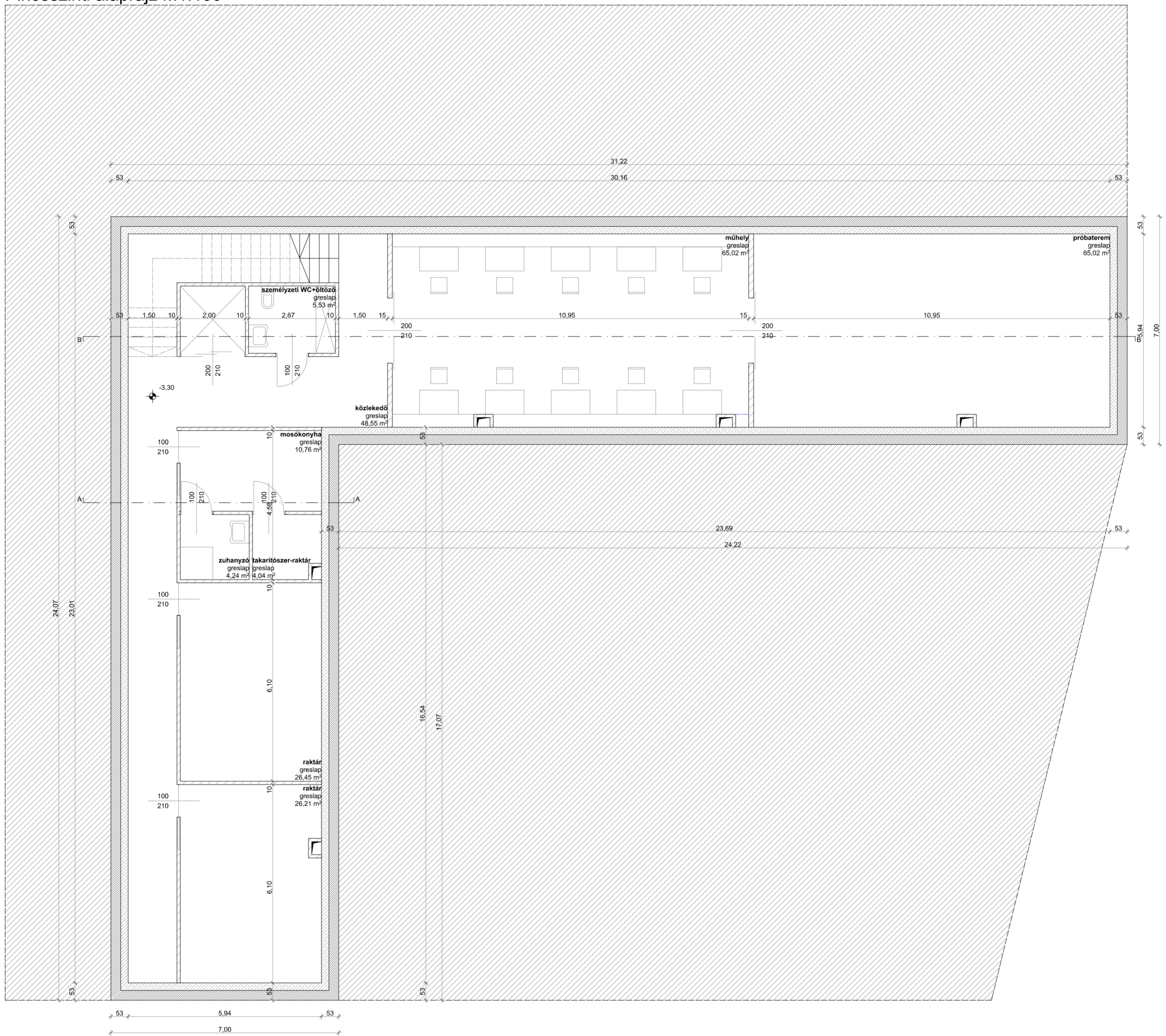
Pincszinti alaprajz M1:100
