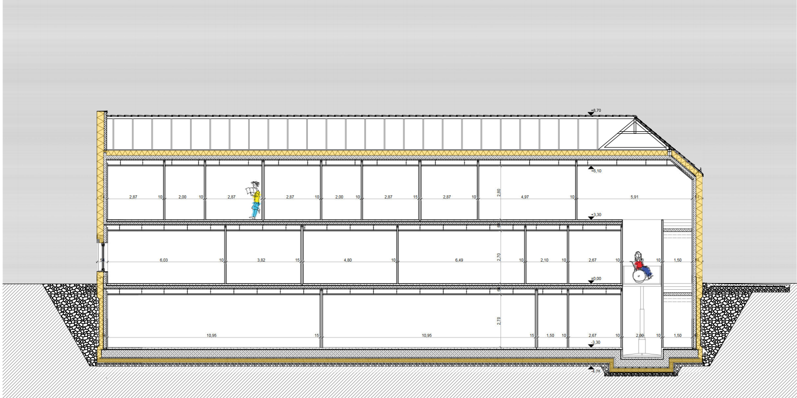
B-B metszet M1:100
