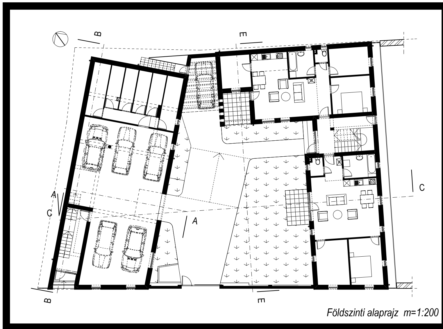
Tata, Kossuth tér 15/b. Terv: Tóbiás Tamás okl. építész
