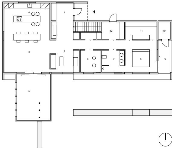
2. FLOOR 1:100
