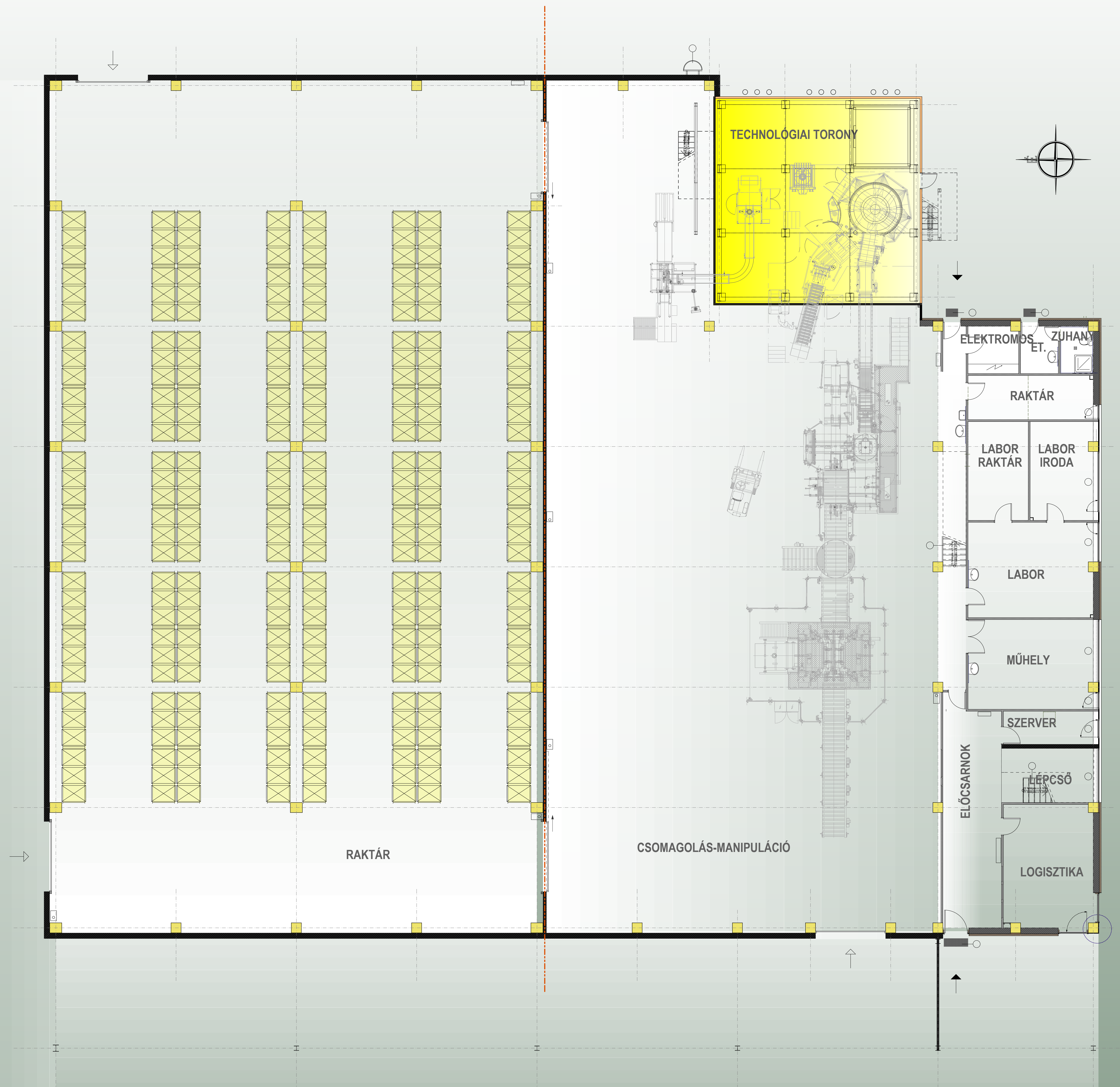
FÖLDSZINTI ALAPRAJZ
