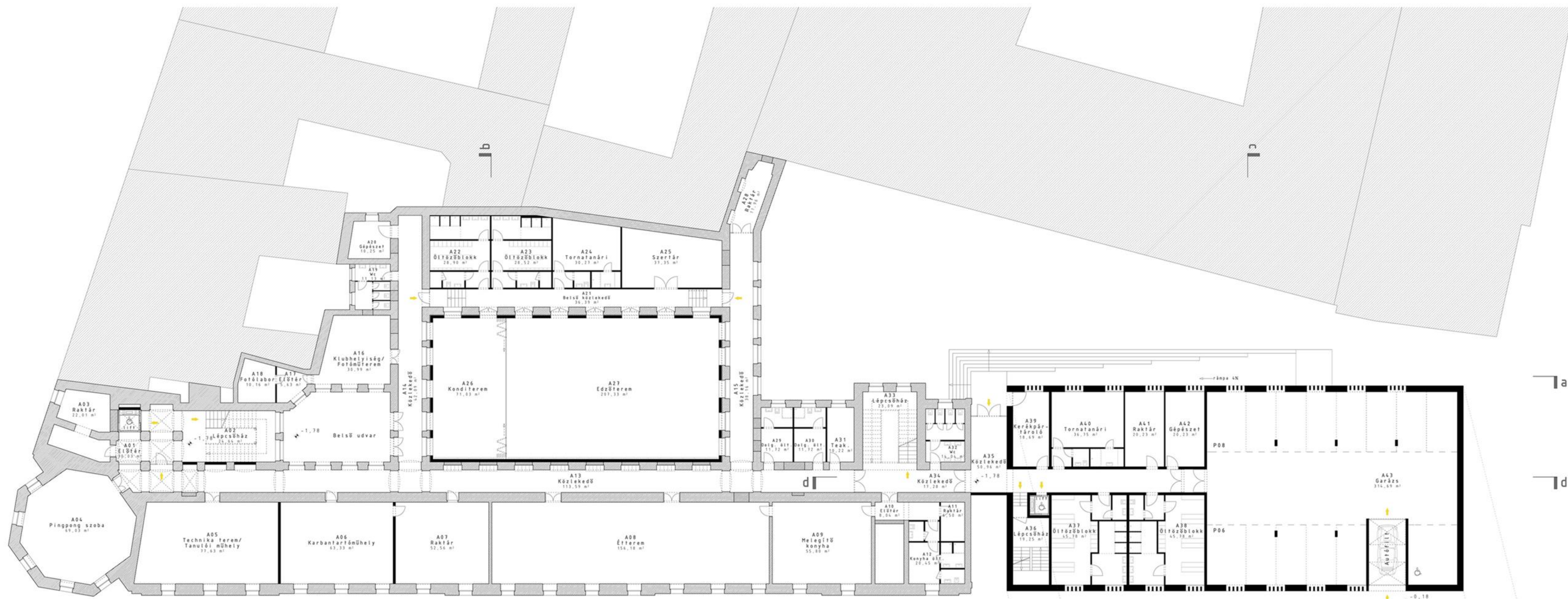
ALAGSORI ALAPRAJZ M1:200
