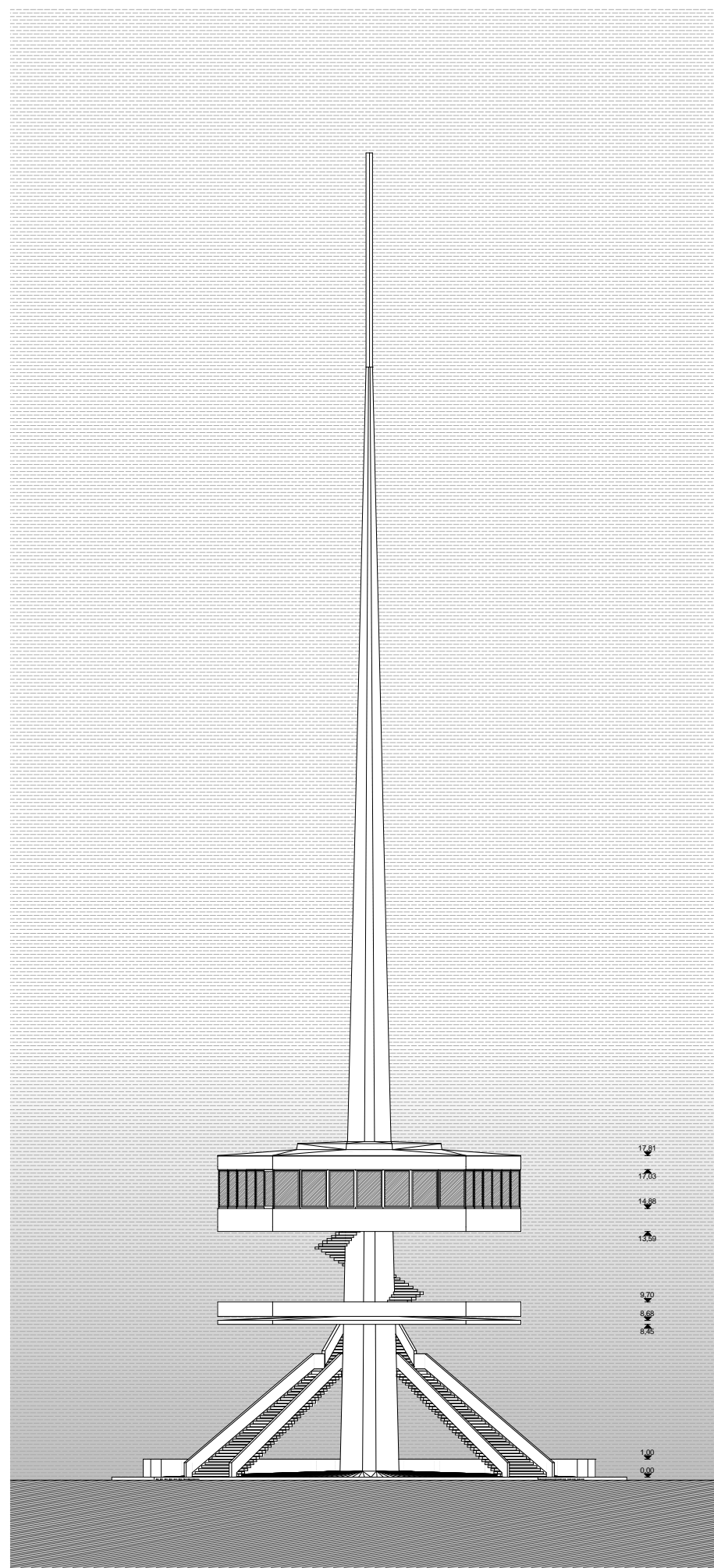
DÉLI HOMLOKZAT
