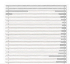
PIHENŐ PAVILON METSZET m=1:50
