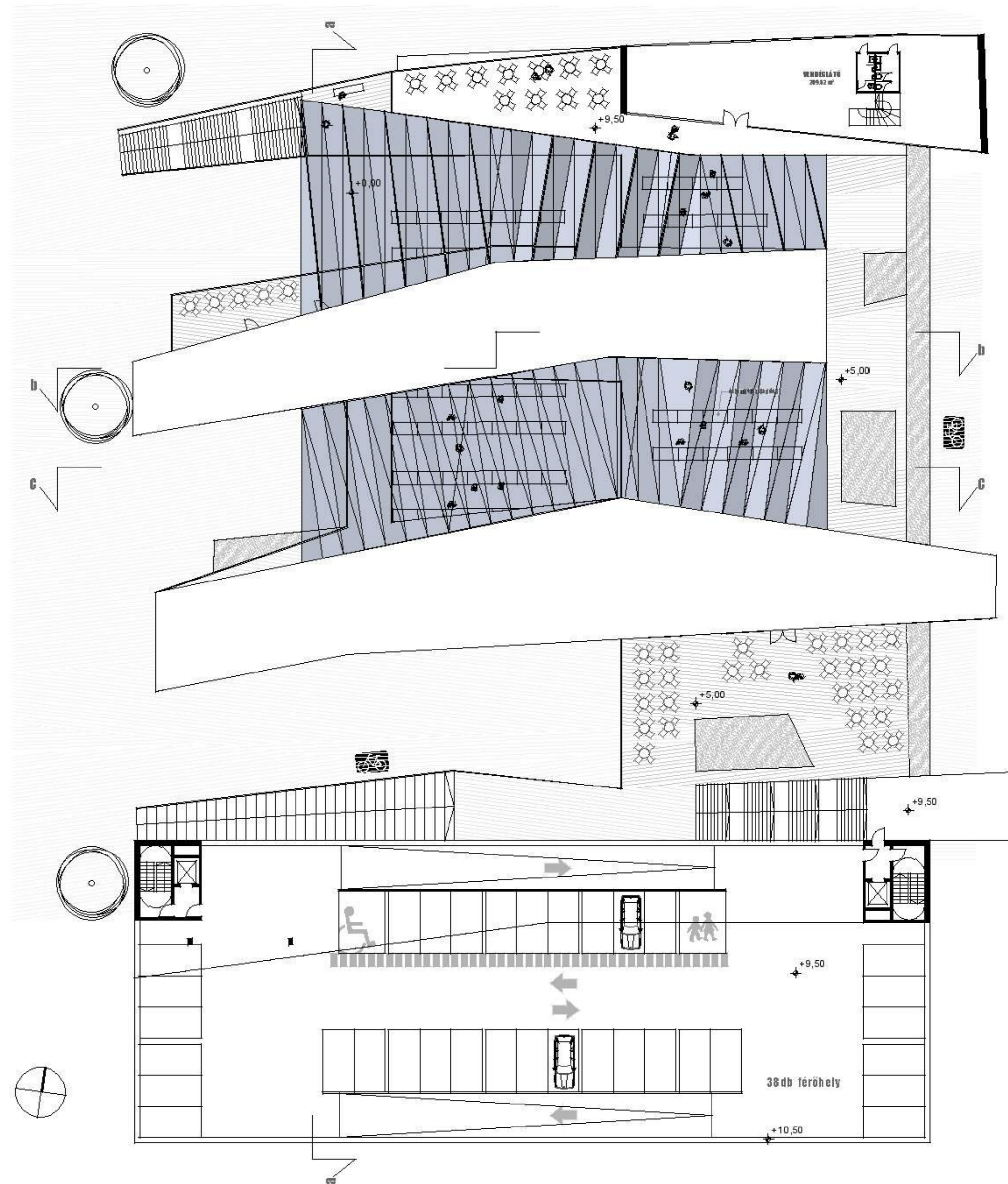
2. SZINT ALAPRAJZA m=1:200
