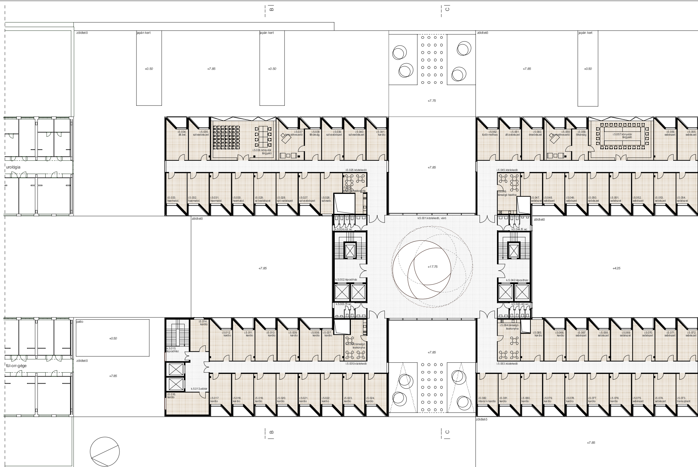
5. emeleti alaprajz
