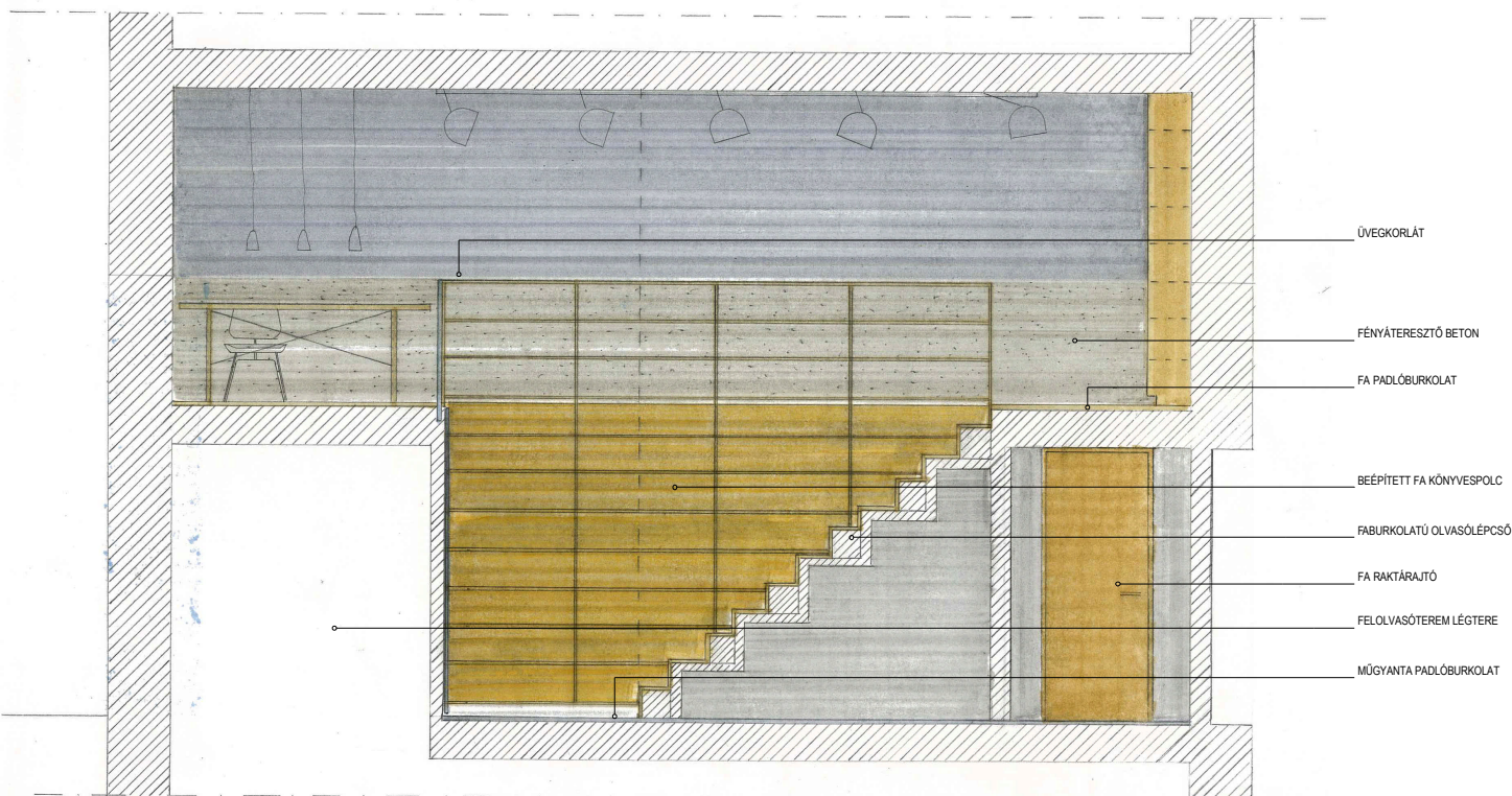
1.1 FALNÉZET M=1:25
