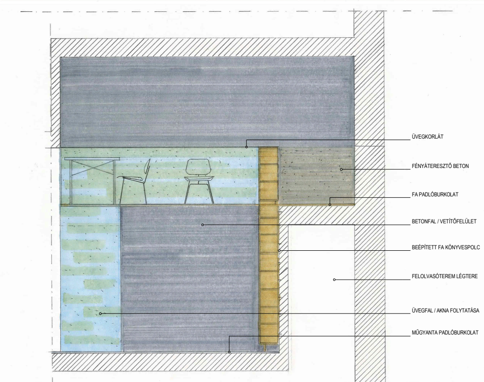
2.2 FALNÉZET M=1:25
