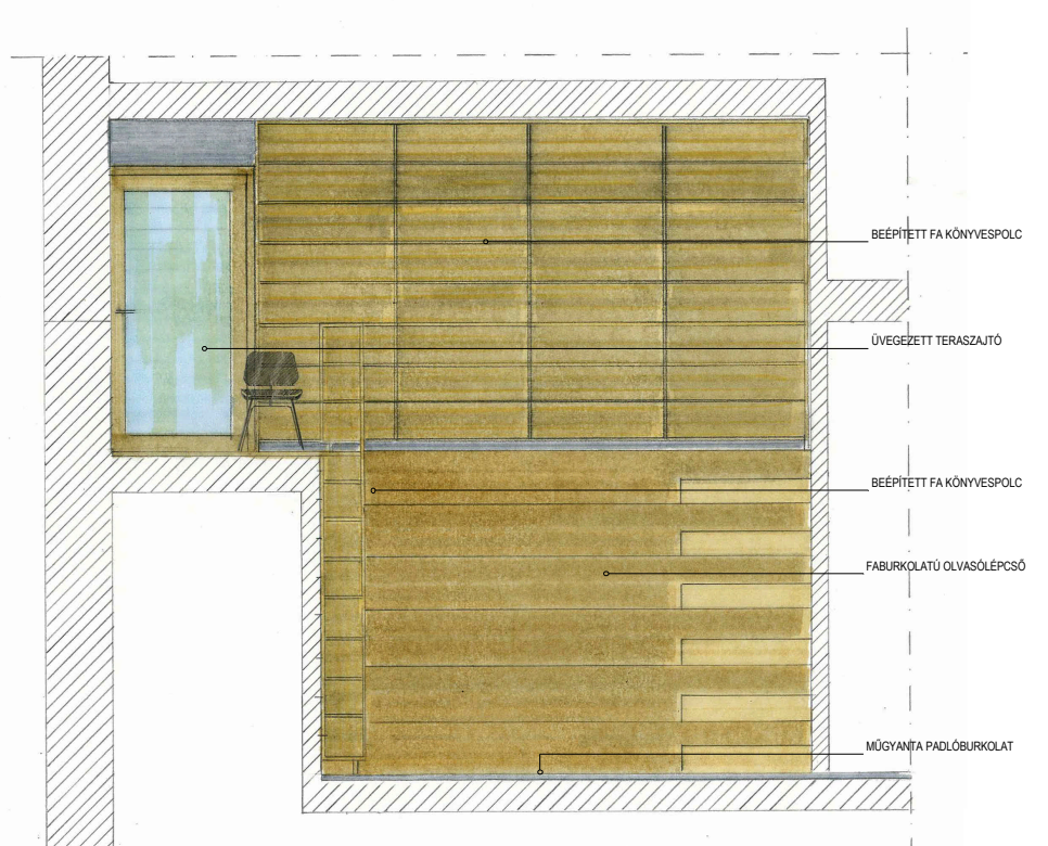
3.3 FALNÉZET M=1:25
