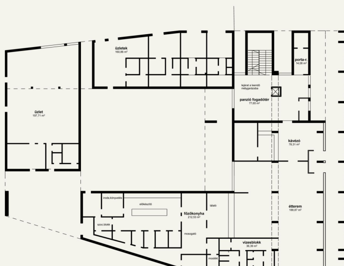
földszinti alaprajz m 1:200
