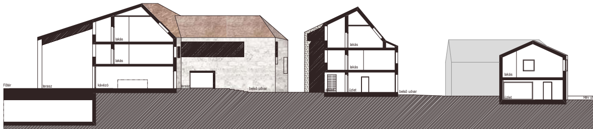
A-A metszet
