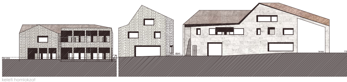
keleti homlokzat
