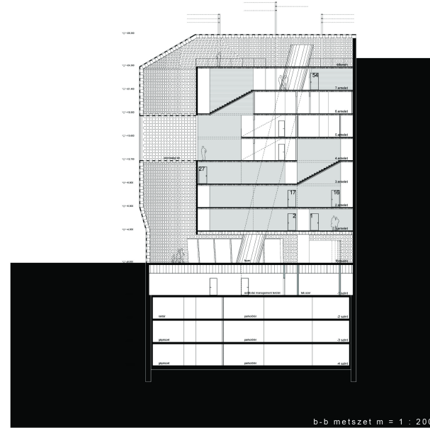
b-b metszet m = 1 : 200
