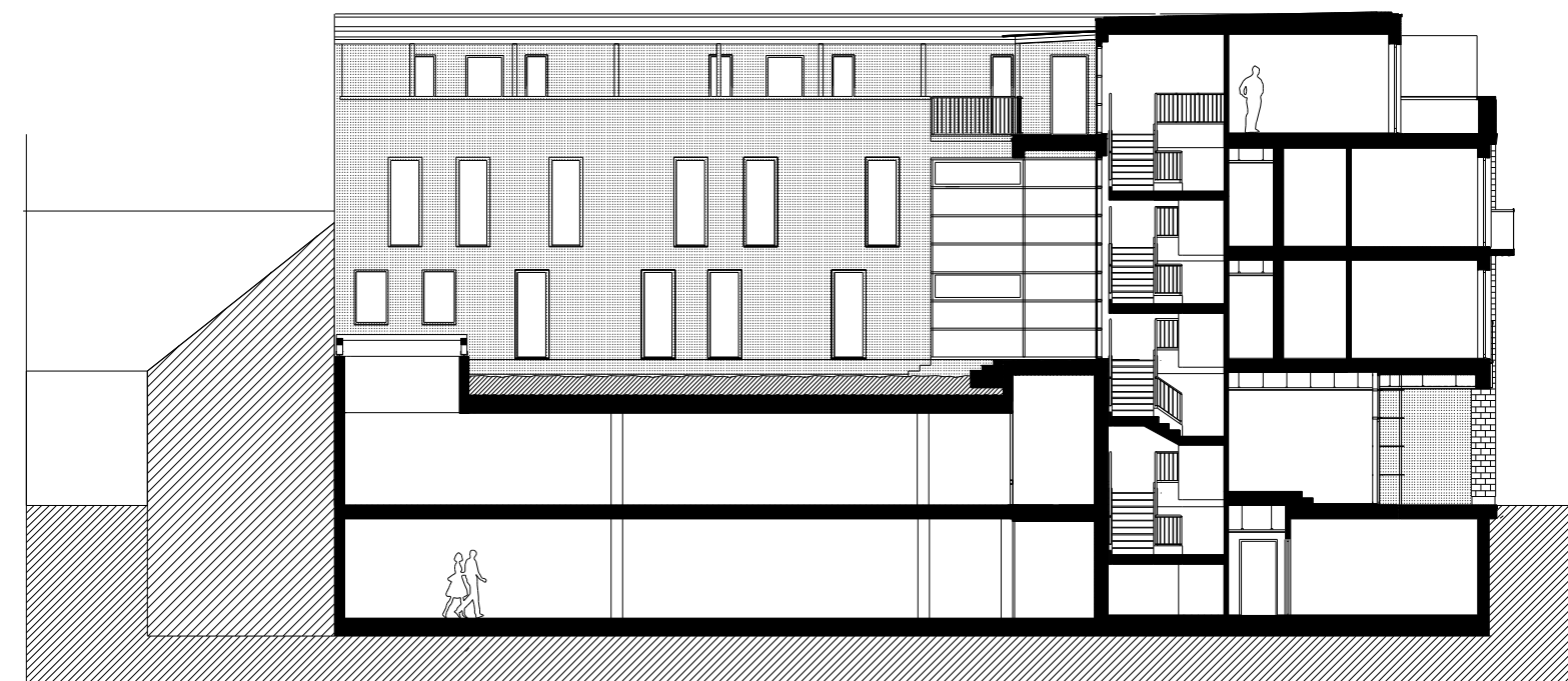
Újpest városközpont . Kemény Gusztáv utcai lakásos társasház, B-B metszet
