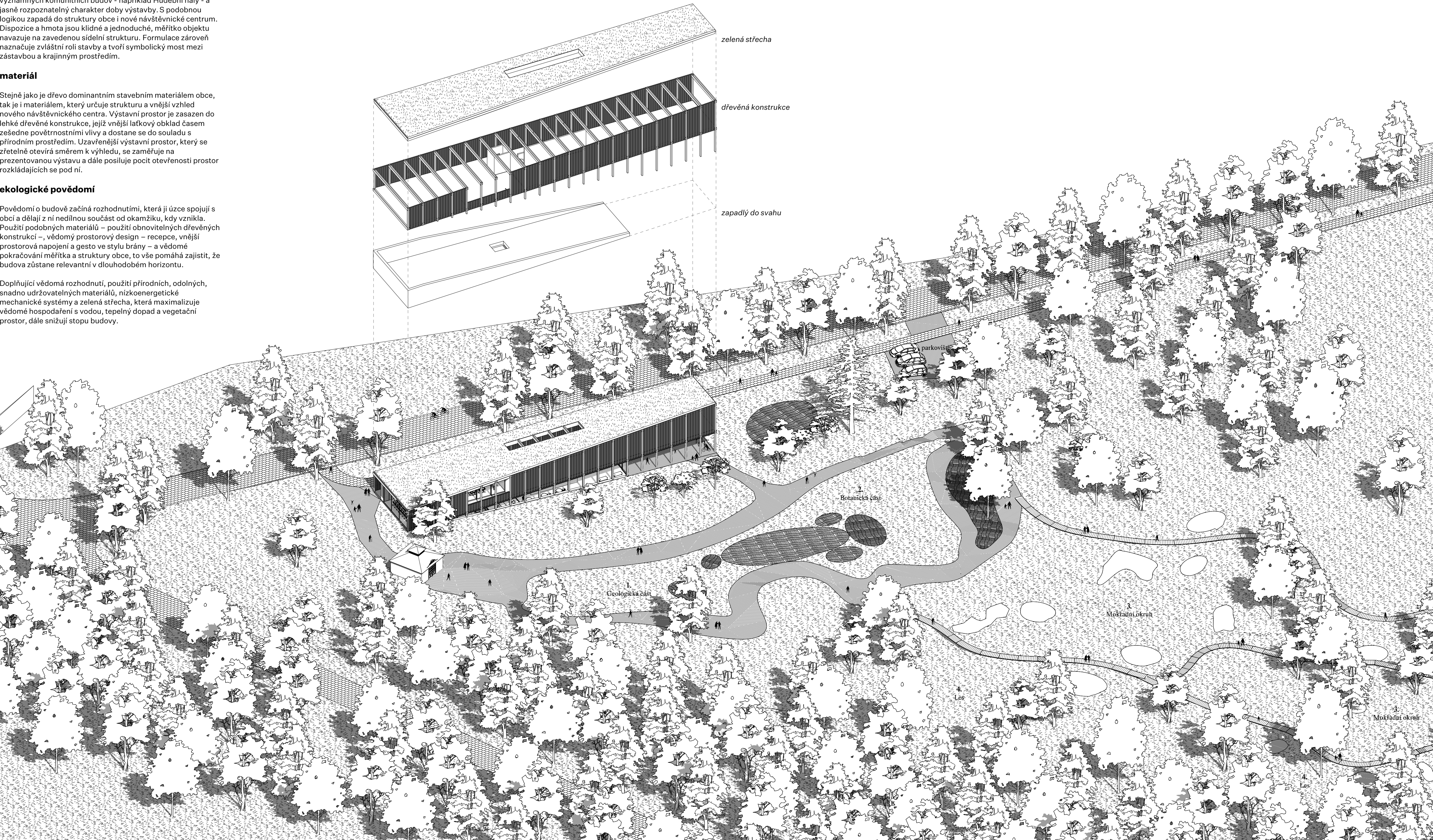
axonometrie
