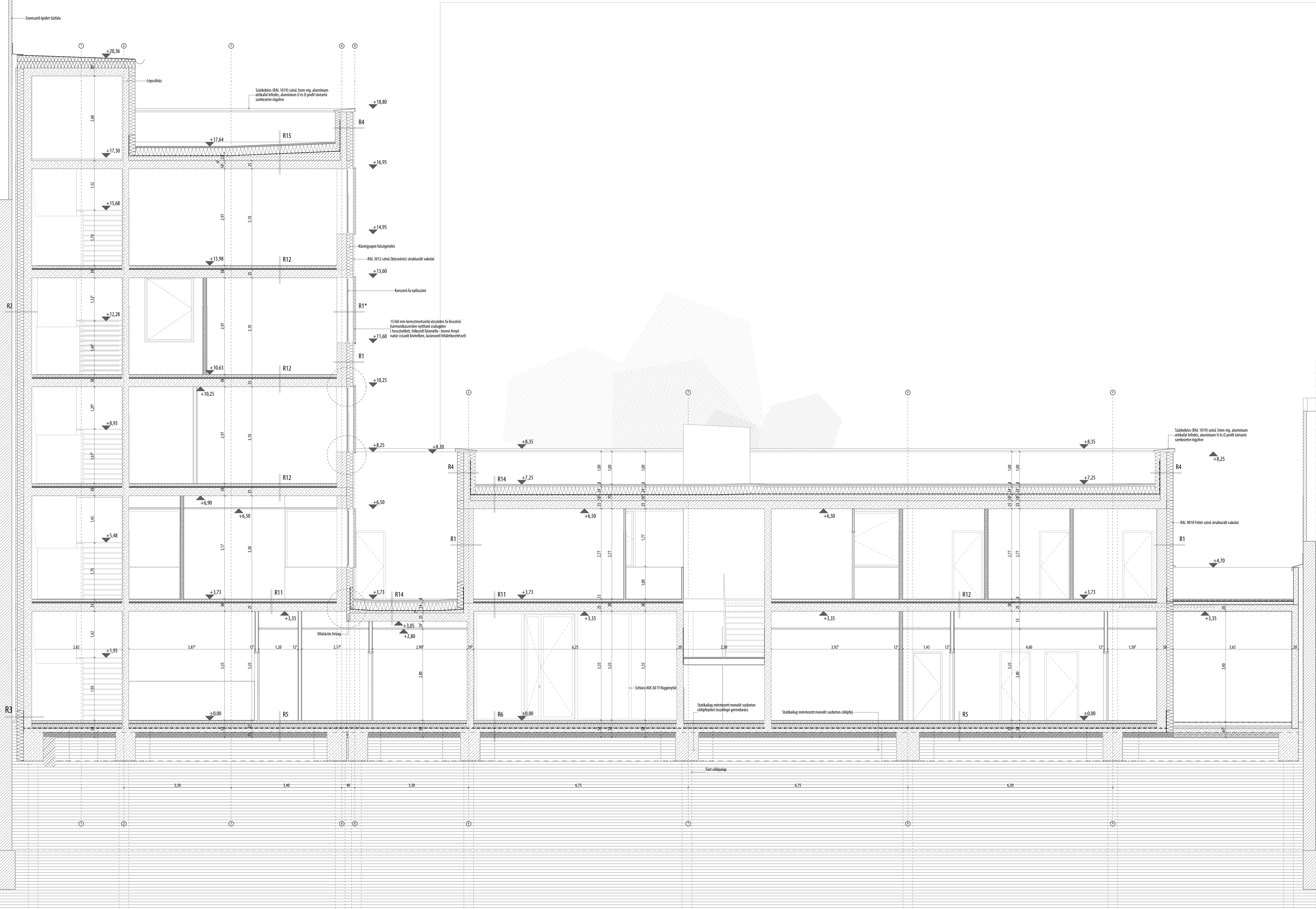
C-C METSZET
