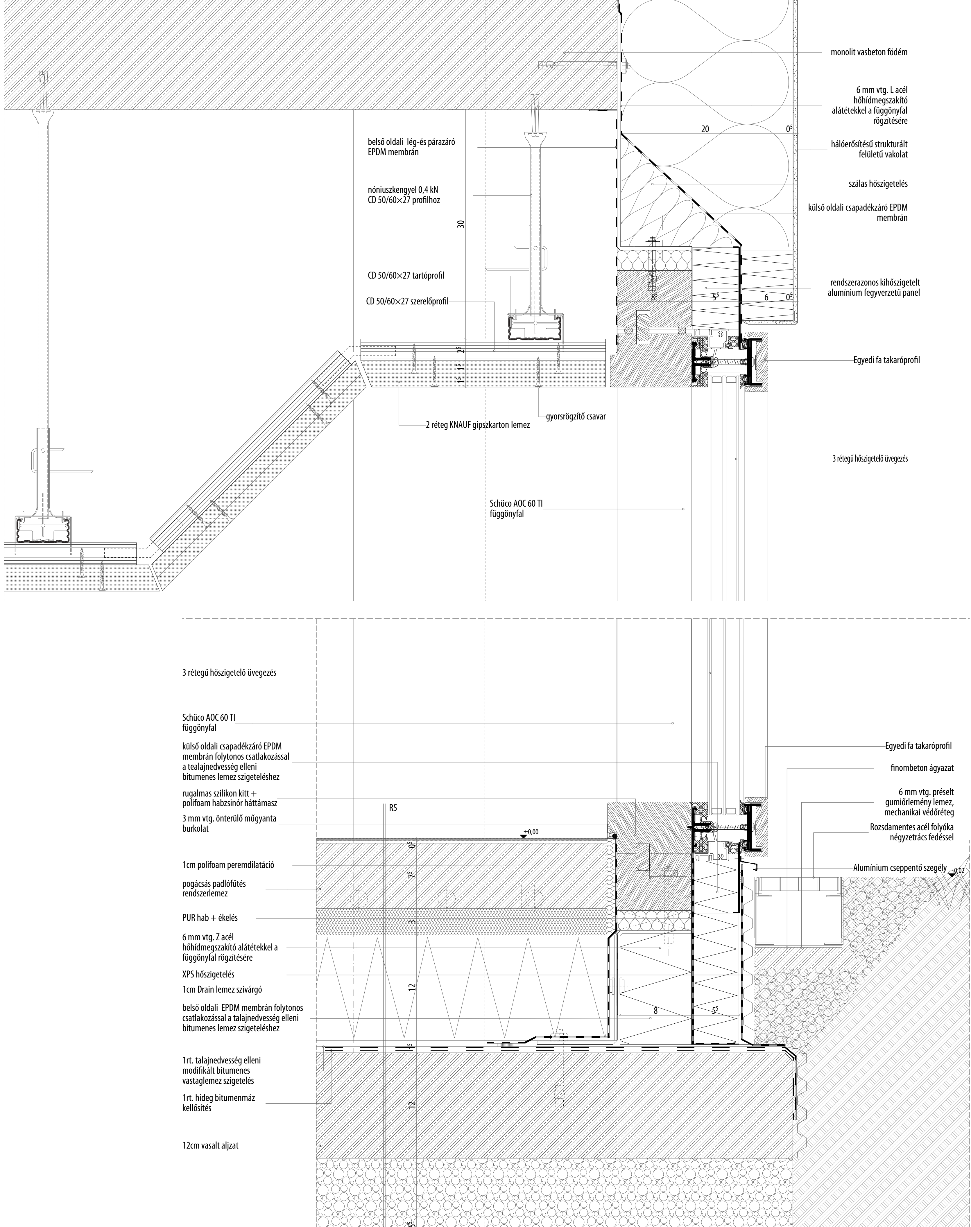
FA BORDAVÁZRA SZERELT FÜGGÖNYFAL BEÉPÍTÉSE
