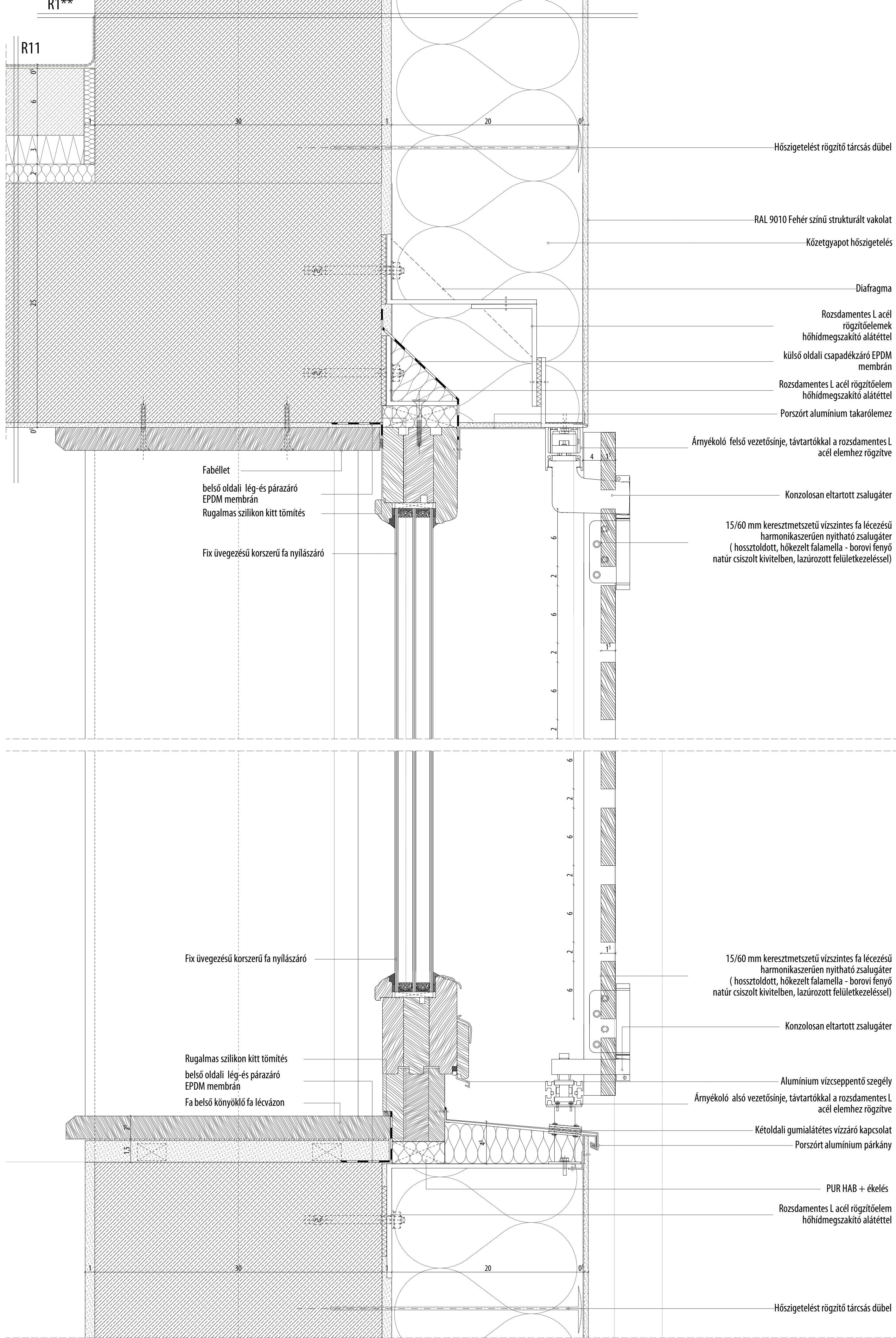
ÁRNYÉKOLÓ ÉS KORSZERŰ FA NYILÁSZÁRÓ BEÉPÍTÉSE
