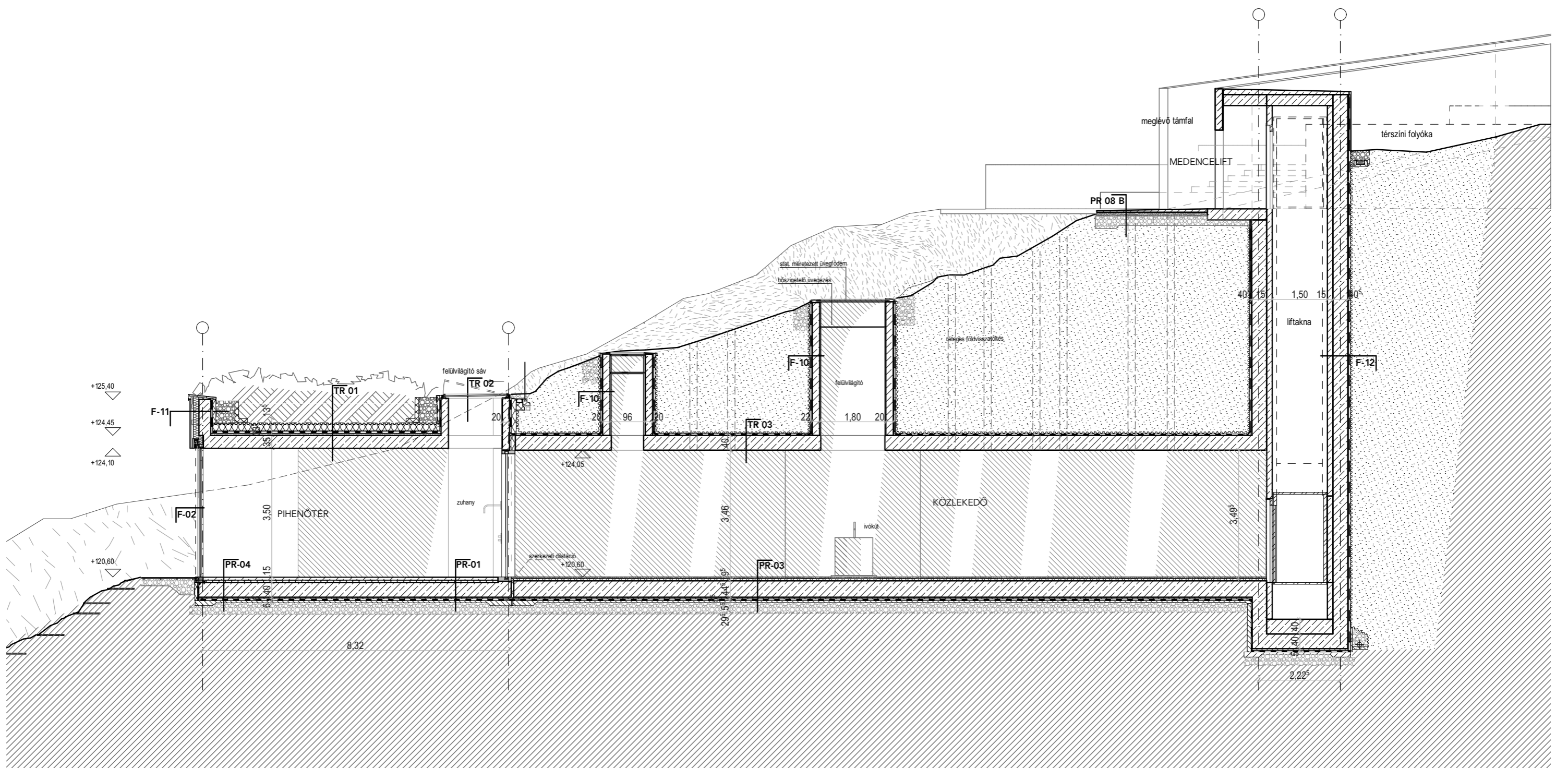
B-B KERESZTMETSZET M=1:300, M=1:50
