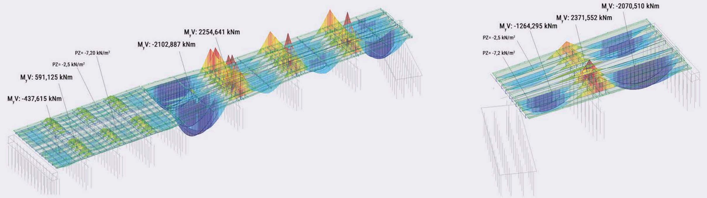
HAJLÍTÓNYOMATÉK ÁBRA A FELSZERKEZETEN TOTAL JÁRMŰ TEHERBŐL - BUDAI OLDALI FELHAJTÓ HÍD BENDING MOMENT UNDER TOTAL TRAFFIC LOAD ON THE SUPERSTRUCTURE - RAMP BRIDGE ON THE BANK (BUDA SIDE)
