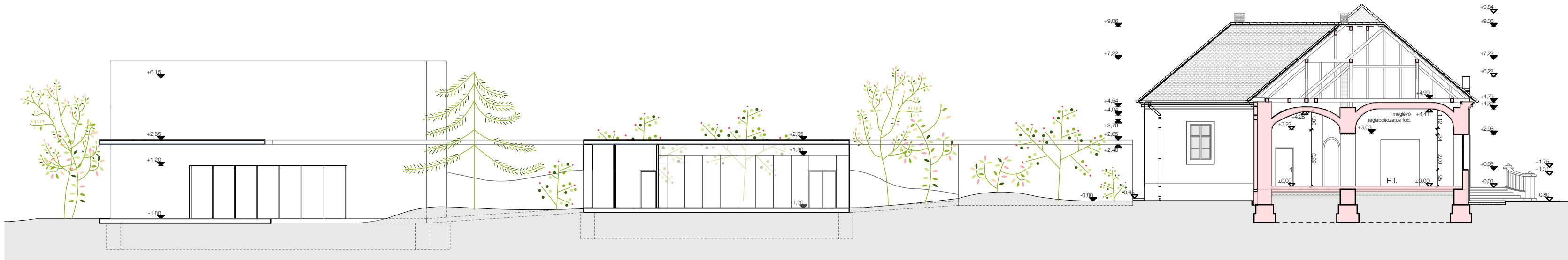
A-A METSZET M 1:200
