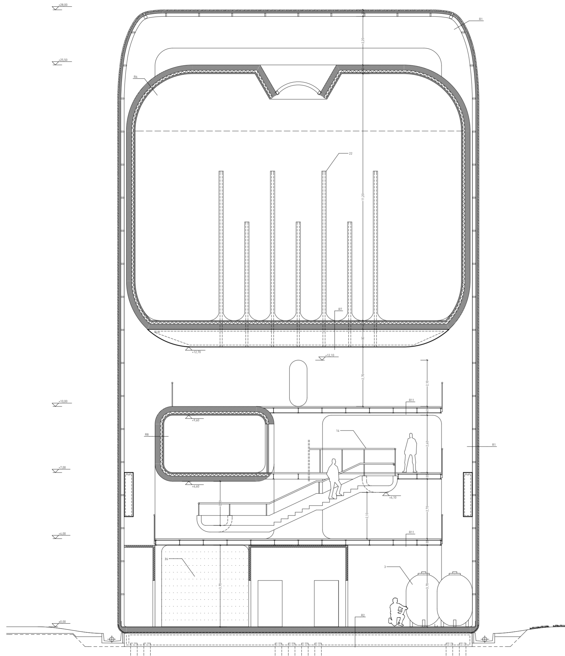
Keresztmetszet 1. / Tervlap 3.1
