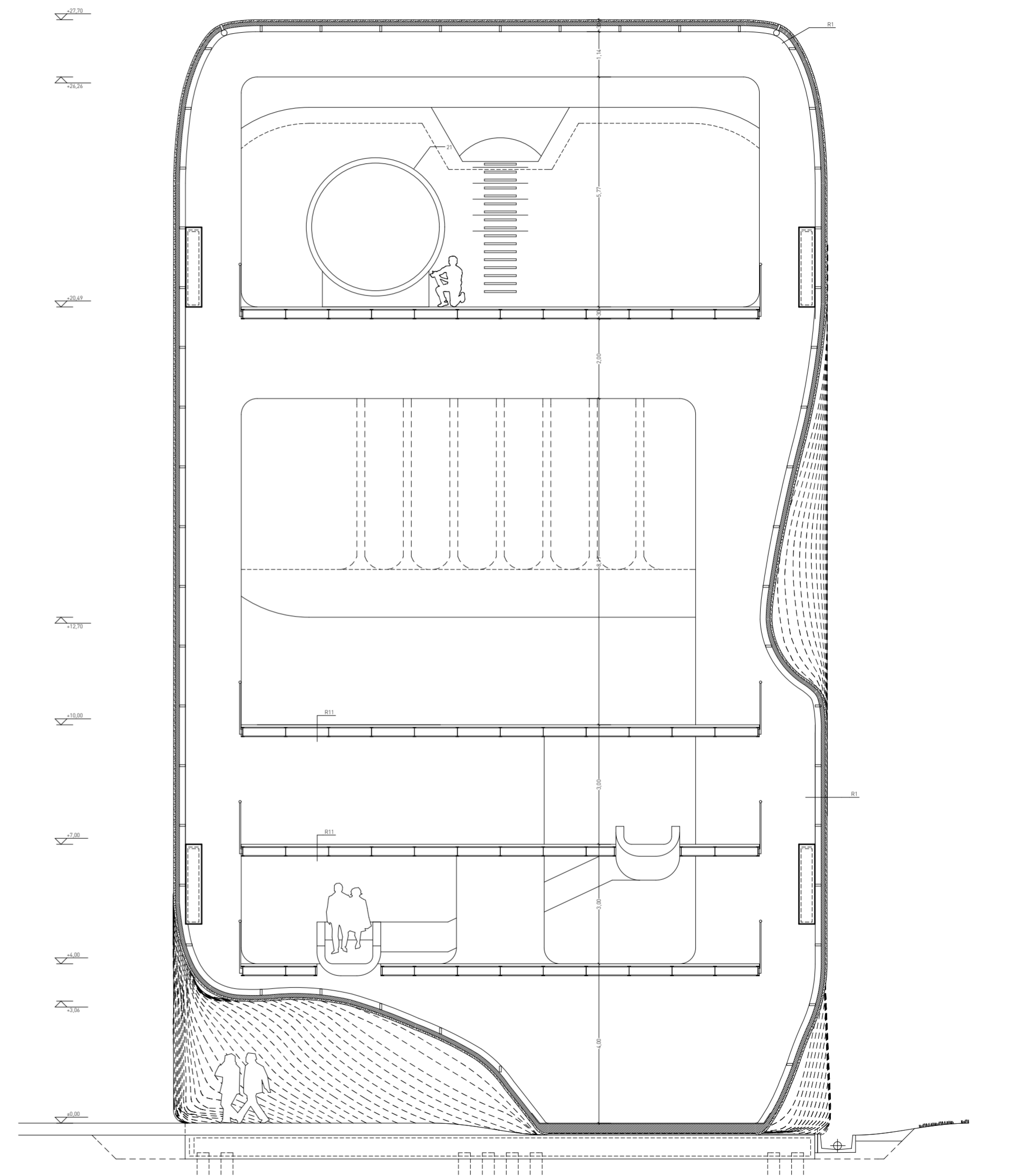
Keresztmetszet 2. / Tervlap 3.2
