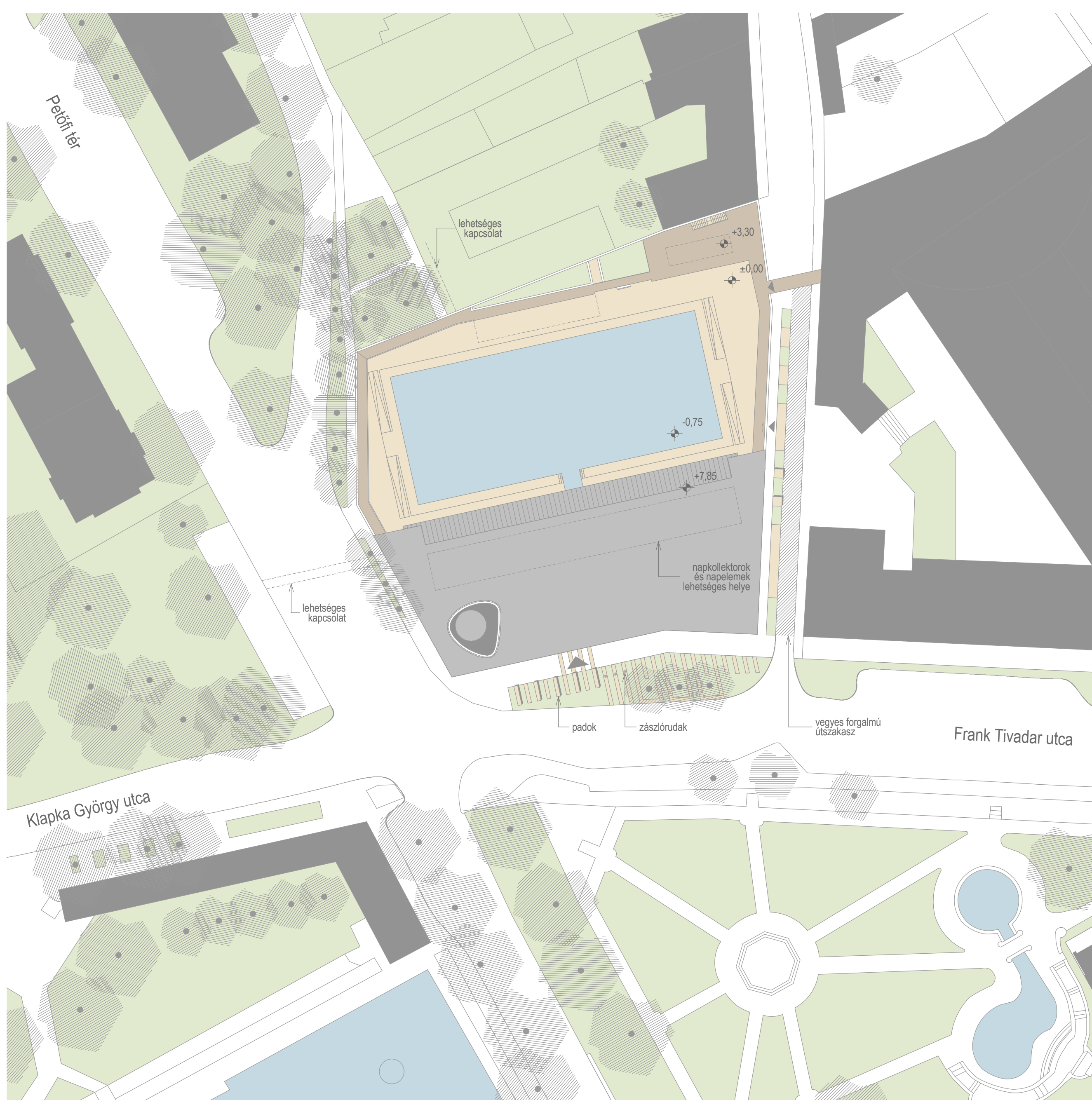
HELYSZÍNRAJZ M 1:500
