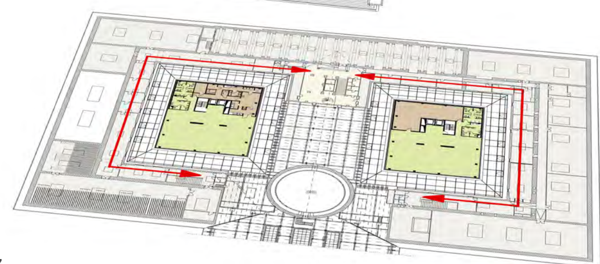
3. EMELETI ALAPRAJZ
