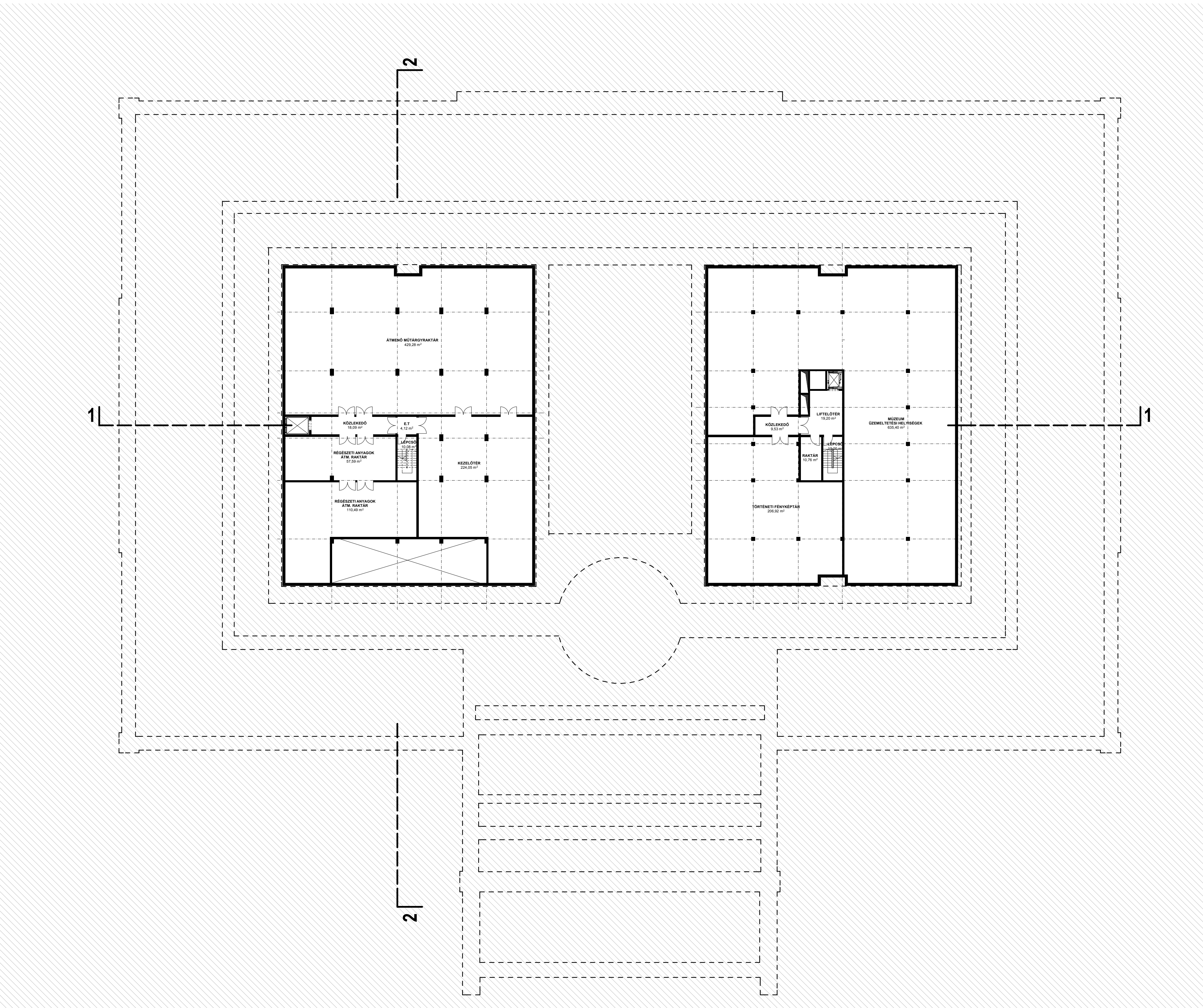
-2. PINCESZINTI ALAPRAJZ
