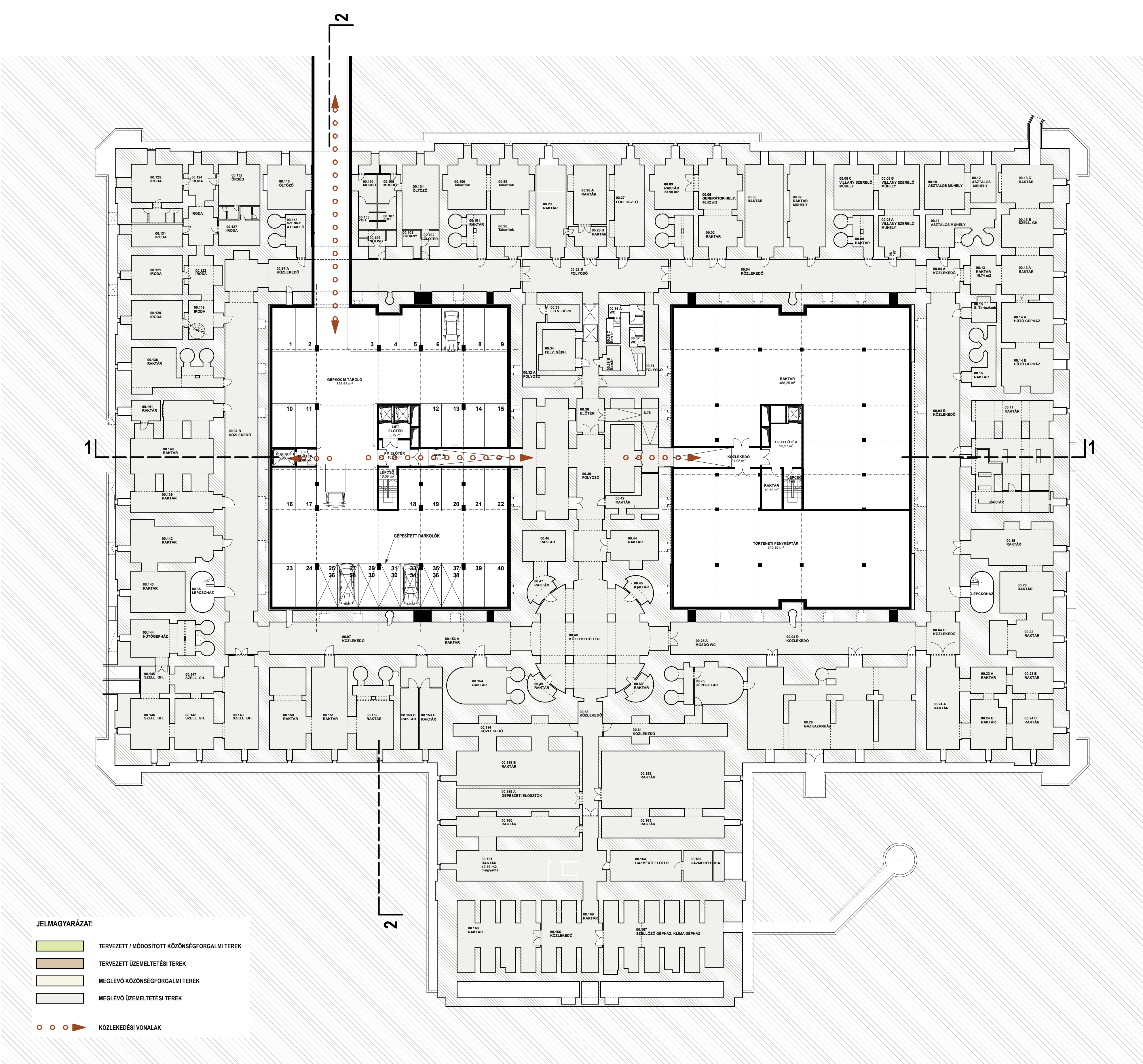
-1. PINCESZINTI ALAPRAJZ
