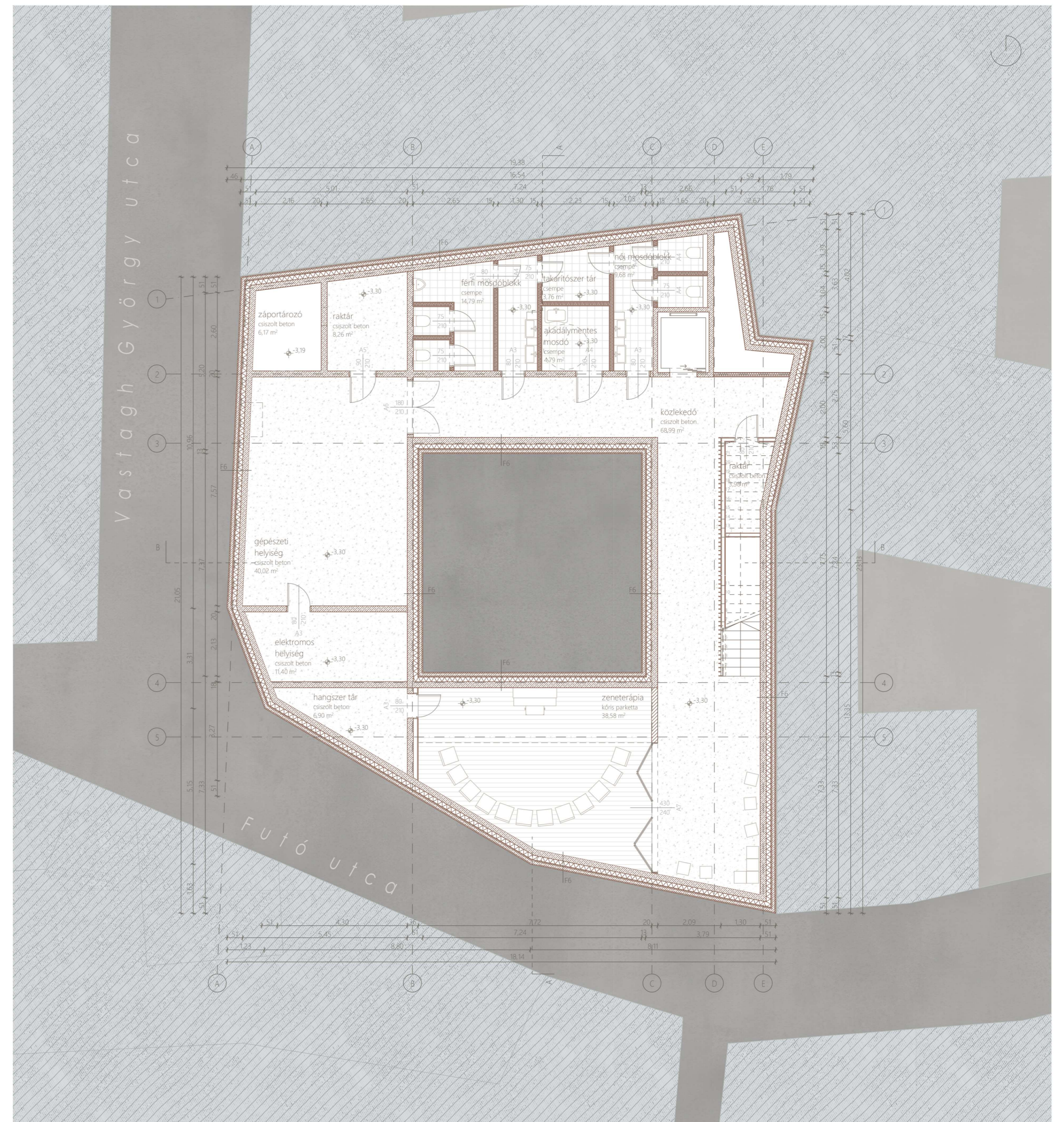
ALAPRAJZ | PINCESZINT
