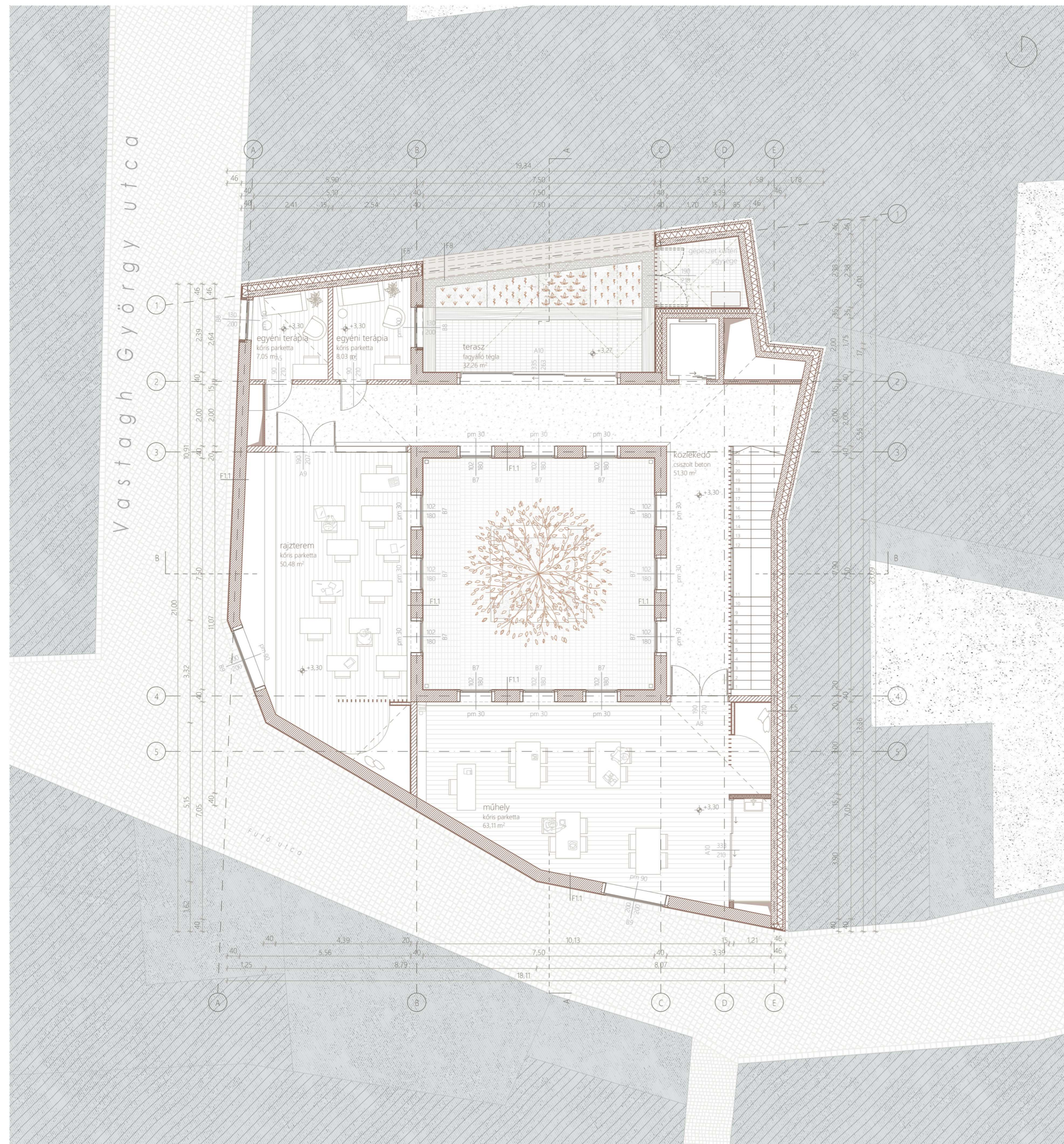
ALAPRAJZ | EMELET
