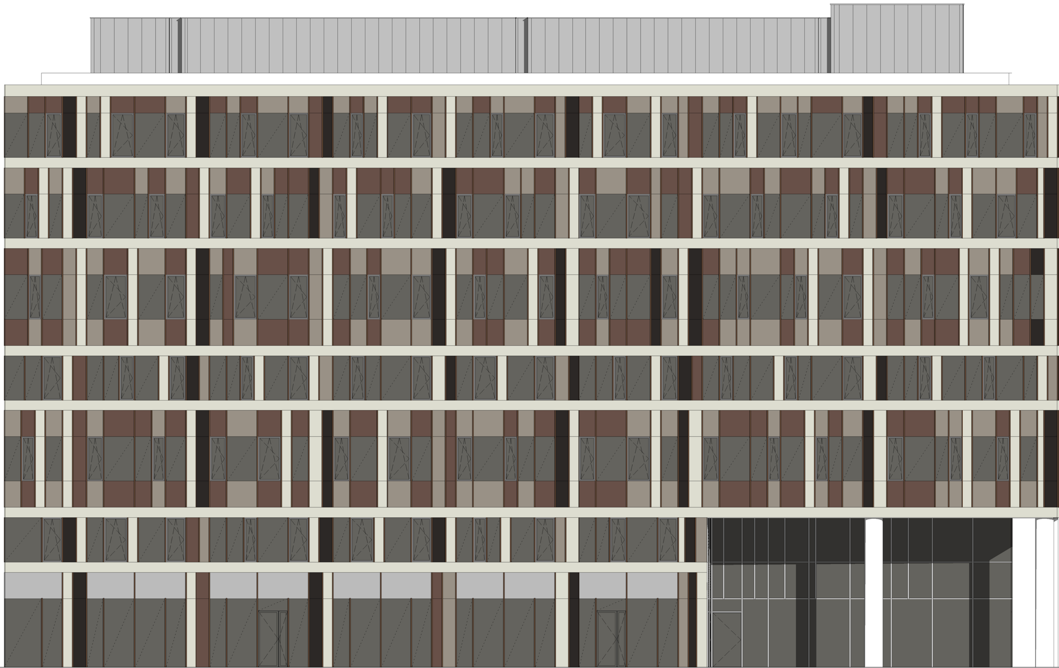
Bence utca Facade M I Scale 1 : 100
