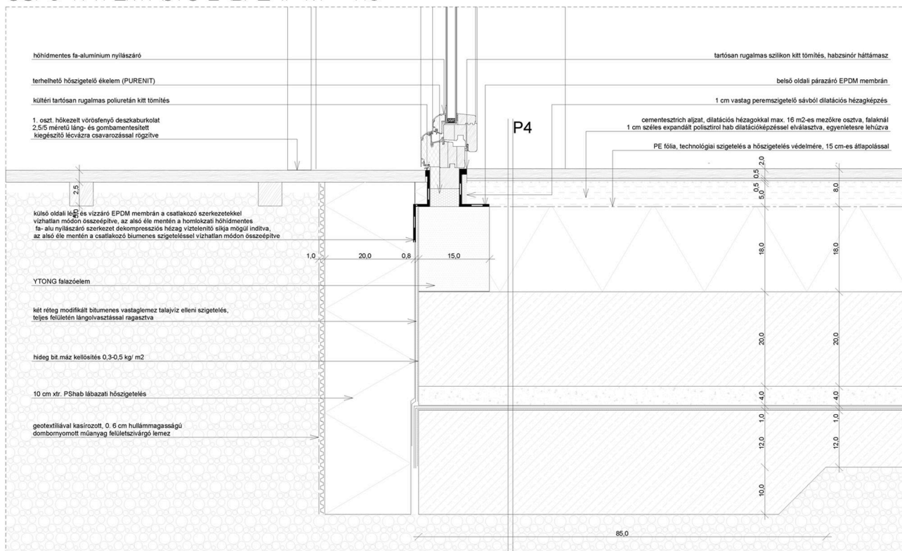
CSP6 FA FÉM AJTÓ LÁBAZAT M = 1:5
