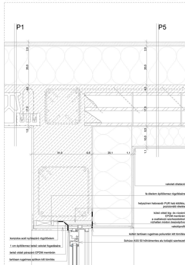
CSP8 TORNÁC TOLÓAJTÓ ALSÓ M = 1:5
