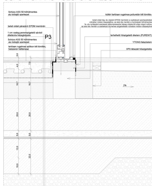
CSP8 TORNÁC TOLÓAJTÓ ALSÓ M = 1:5
