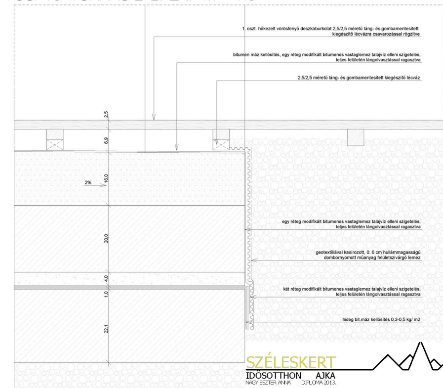
CSP10 TORNÁC LÁBAZAT M = 1:5
