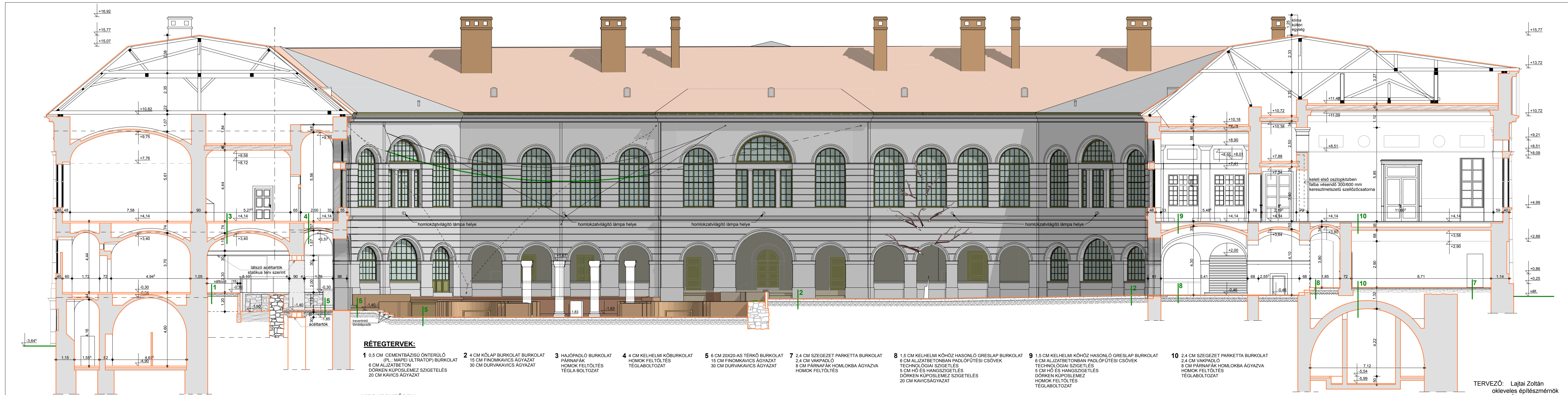
TERVEZETT B-B METSZET ÉS BELSŐ HOMLOKZAT M=1:100
